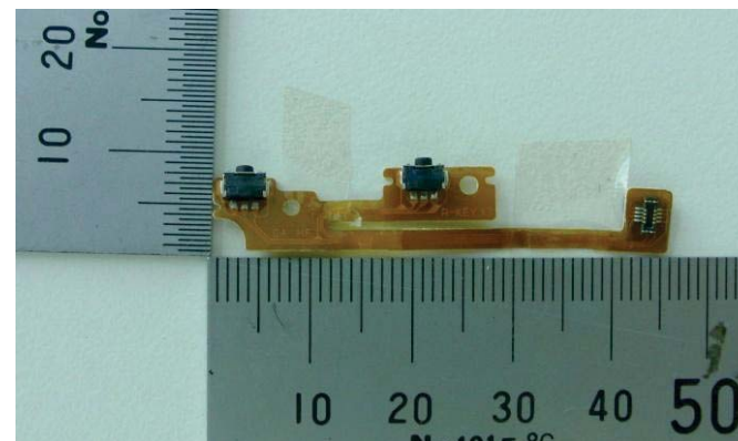
AYS-KTR-FPC/RKEY/*/0X-C0
