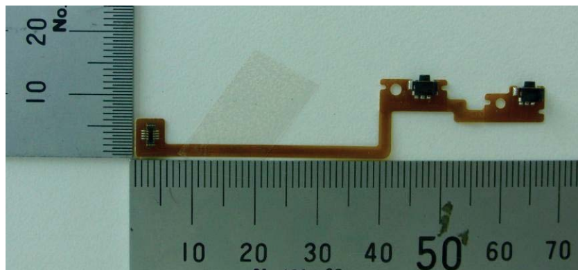
AYS-KTR-FPC/LKEY/*/0X-C0
