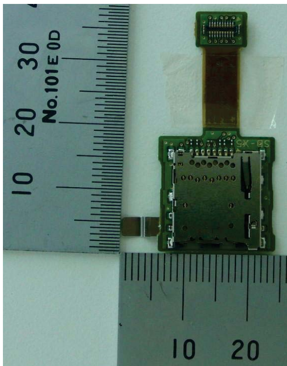
AYS-KTR-RFPCB/SD/0X-C0
