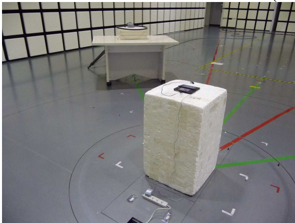
Rear (30-1000MHz)
