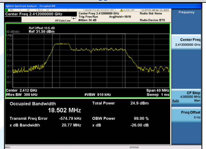
IEEE 802.11ax_Channel 1_20MHz_Antenna 1_RU&amp;Index 52RU37
