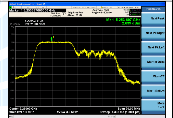
IEEE 802.11ax_Channel 52_20MHz_Antenna 2_RU&Index 106RU53
