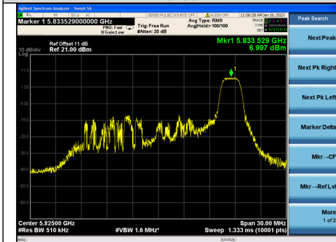
IEEE 802.11ax_Channel 165_20MHz_Antenna 2_RU&amp;Index 26RU8
