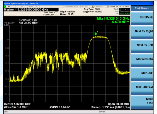
IEEE 802.11ax_Channel 64_20MHz_Antenna 2_RU&amp;Index 52RU40
