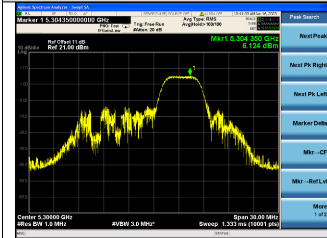
IEEE 802.11ax_Channel 60_20MHz_Antenna 2_RU&amp;Index 52RU39
