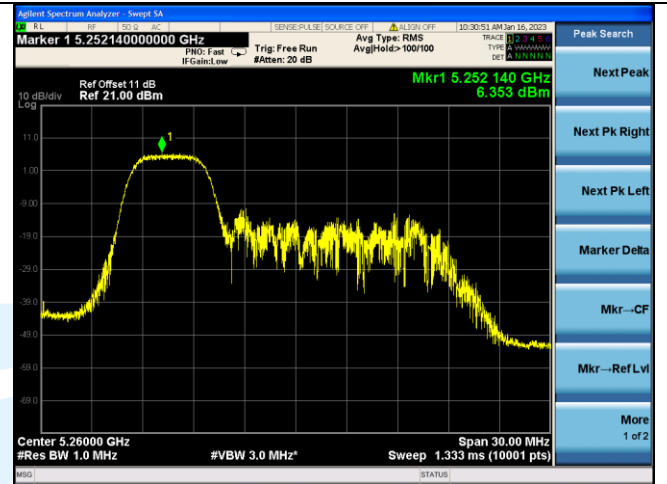
IEEE 802.11ax_Channel 52_20MHz_Antenna 2_RU&amp;Index 52RU37
