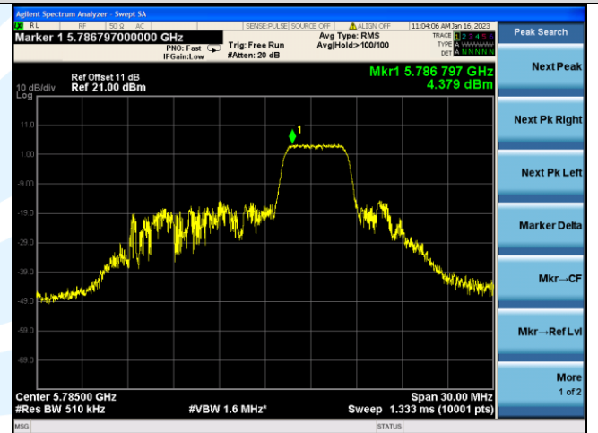
IEEE 802.11ax_Channel 157_20MHz_Antenna 2_RU&amp;Index 52RU39
