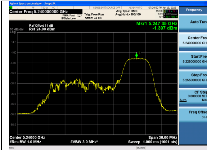
IEEE 802.11ax_Channel 48_20MHz_Antenna 2_RU&amp;Index 52RU40
