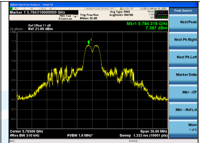
IEEE 802.11ax_Channel 157_20MHz_Antenna 2_RU&amp;Index 26RU4
