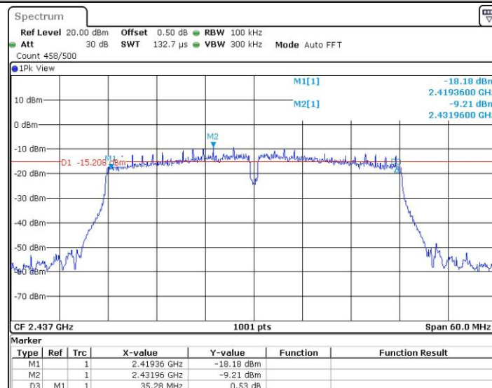
11N40SISO_ANT0_2437
