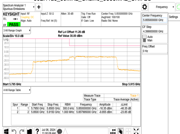
802.11ac_80MHz_Chain0_5855MHz_UNII 2C
