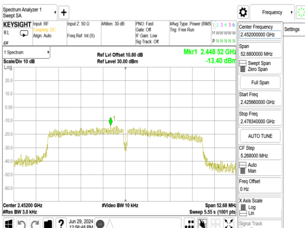
802.11n_40MHz_Chain0_2452MHz
