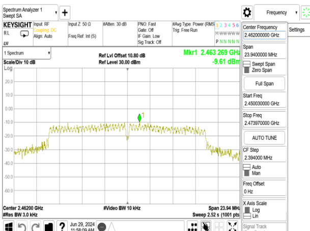
802.11g_20MHz_Chain0_2462MHz
