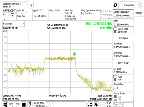
802.11ax_20MHz_Chain1_2462MHz_RU26_8
