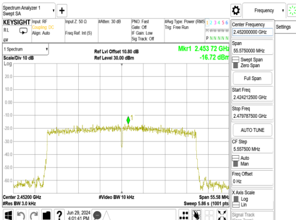
802.11ax_40MHz_Chain1_2452MHz
