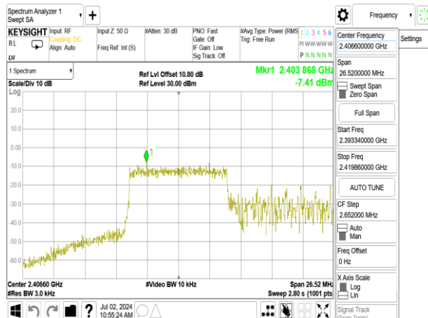
802.11ax_20MHz_Chain1_2412MHz_RU26_0
