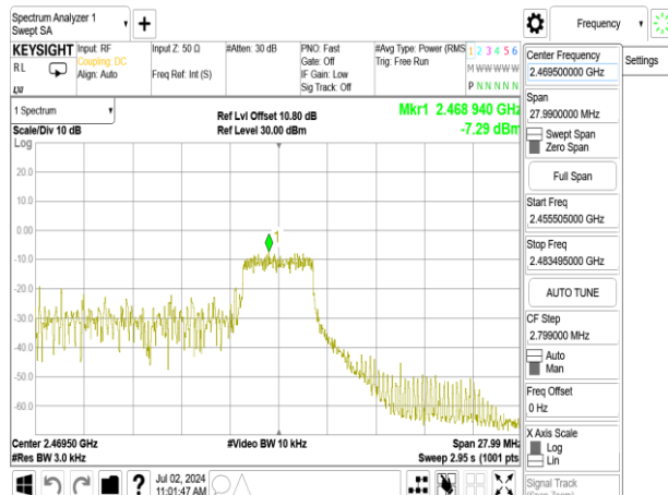
802.11ax_20MHz_Chain1_2462MHz_RU52_40
