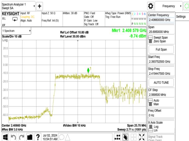
802.11ax_20MHz_Chain0_2412MHz_RU26_0
