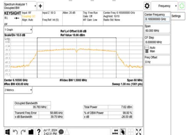
802.11n_40MHz_Chain0_6165MHz
