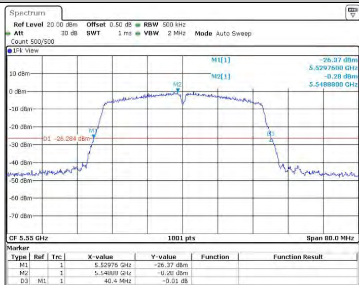
11AC40MIMO_Ant1_5550
