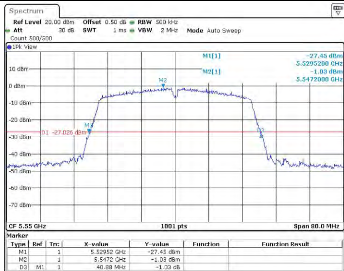
11AC40MIMO_Ant1_5550
