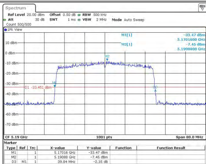
11AX40MIMO_Ant2_5190
