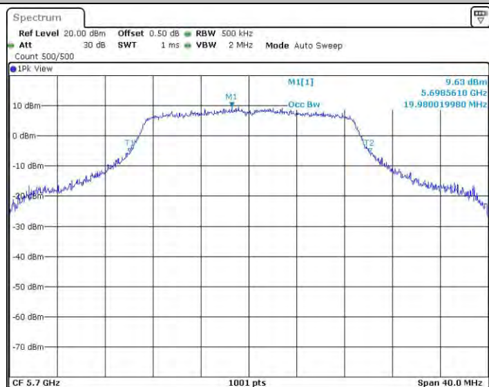
11N20SISO_Ant2_5700
