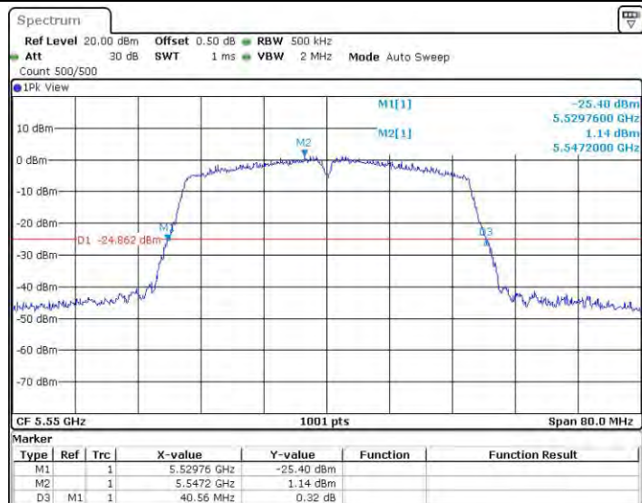
11N40MIMO_Ant2_5550
