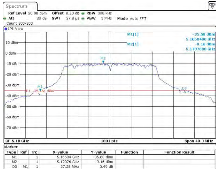
11AC20MIMO_Ant1_5180
