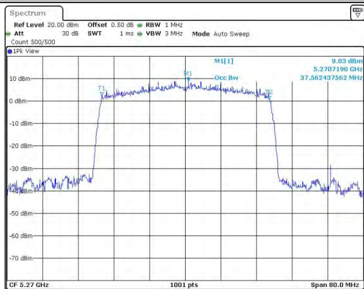
11AX40SISO_Ant1_5270
