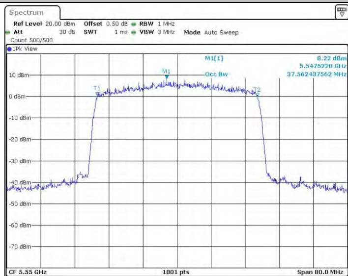
11AX40SISO_Ant2_5550
