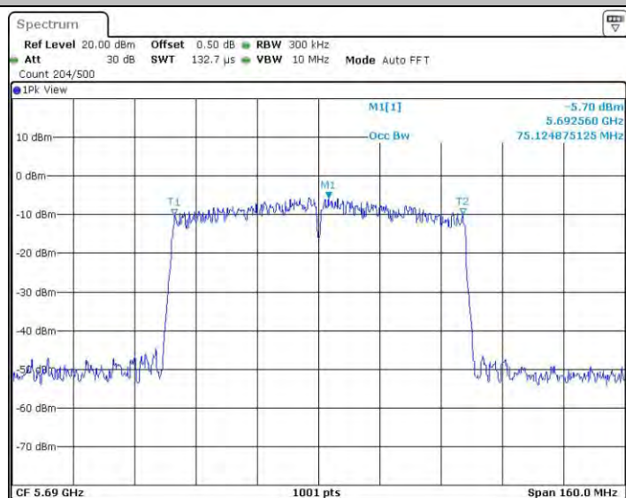
11AC80MIMO_Ant2_5690
