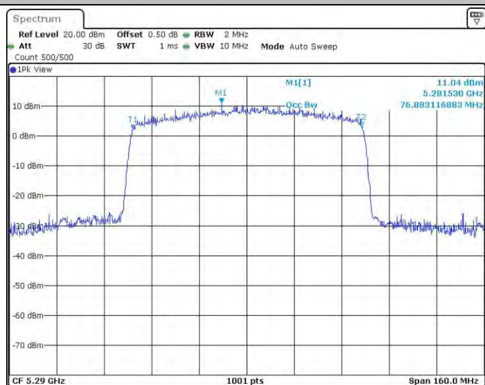
11AX80SISO_Ant1_5290
