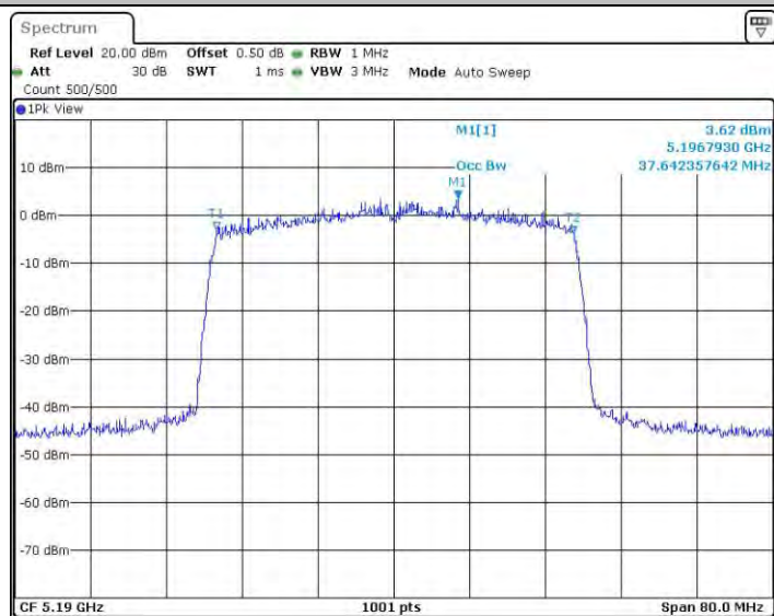
11AX40SISO_Ant2_5190
