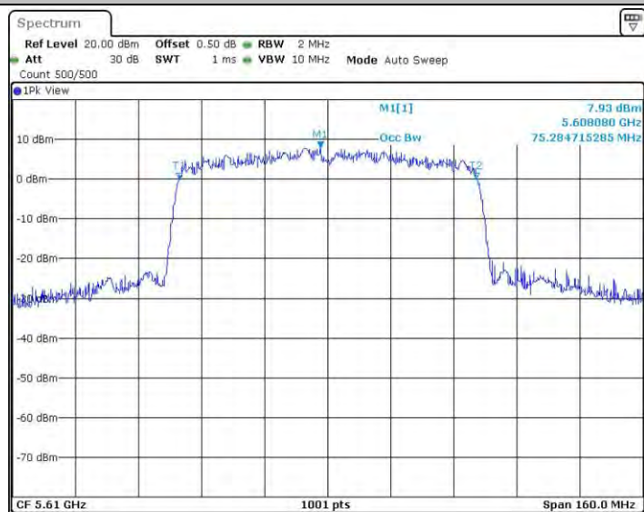
11AC80SISO_Ant1_5610
