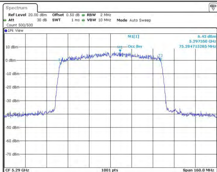
11AC80MIMO_Ant2_5290
