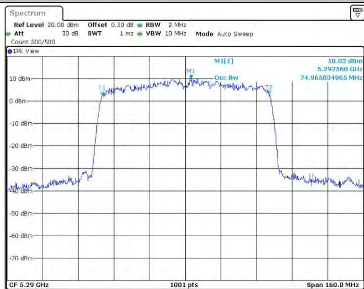
11AC80SISO_Ant2_5290
