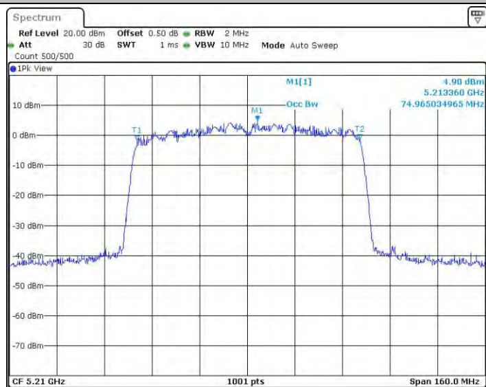
11AC80SISO_Ant2_5210
