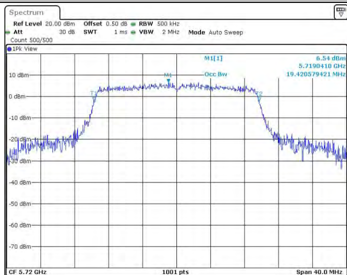
11AX20SISO_Ant1_5720
