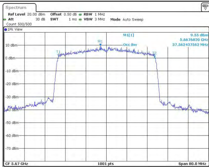
11AX40SISO_Ant2_5670
