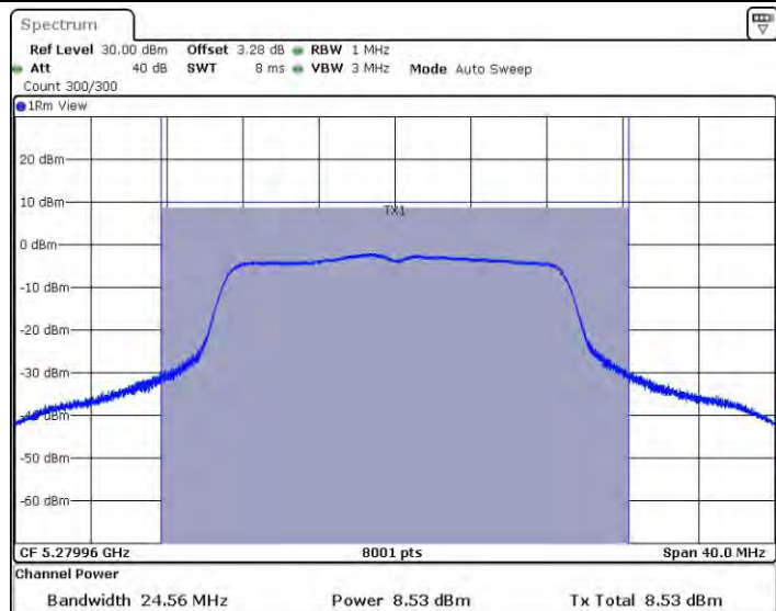
11AC20MIMO_Ant1_5280
