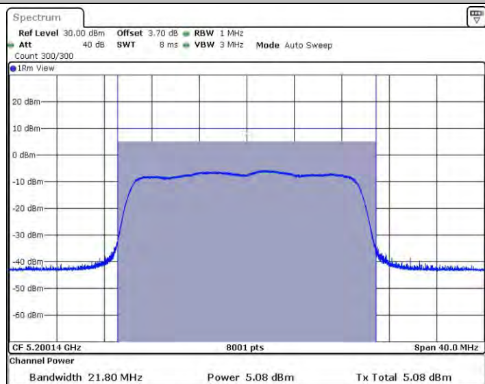
11AX20SISO_Ant2_5200
