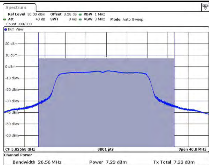
11AC20MIMO_Ant2_5825
