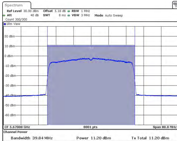
11AX40SISO_Ant2_5670
