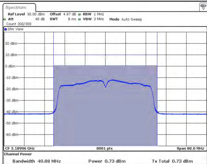
11AC40MIMO_Ant1_5190
