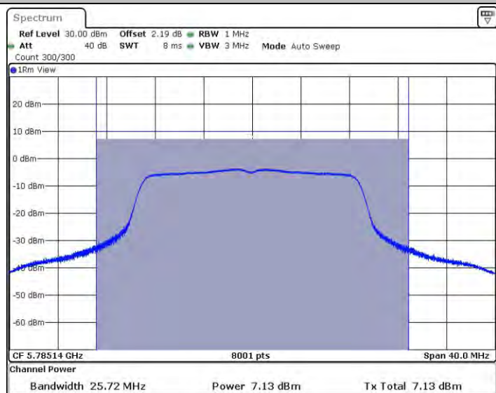
11N20MIMO_Ant1_5785
