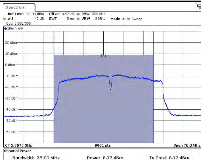
11AC40MIMO_Ant2_5710_UNII-2C
