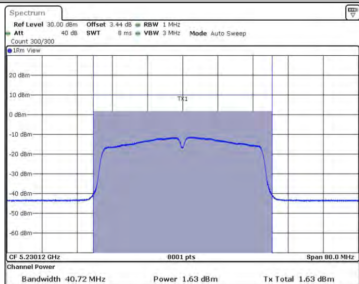
11N40MIMO_Ant1_5230
