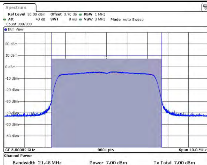
11AX20MIMO_Ant2_5580
