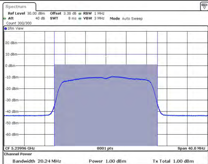
11AC20MIMO_Ant2_5240
