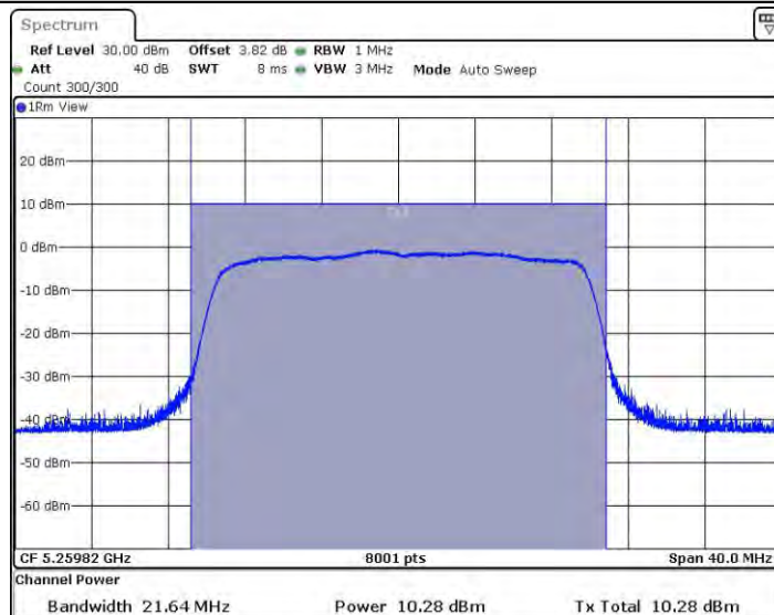
11AX20SISO_Ant2_5260
