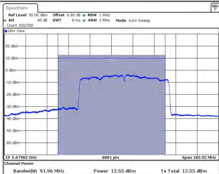
11AC80SISO_Ant1_5690_UNII-2C
