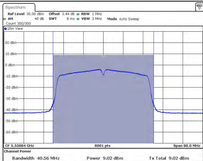
11N40MIMO_Ant2_5550
