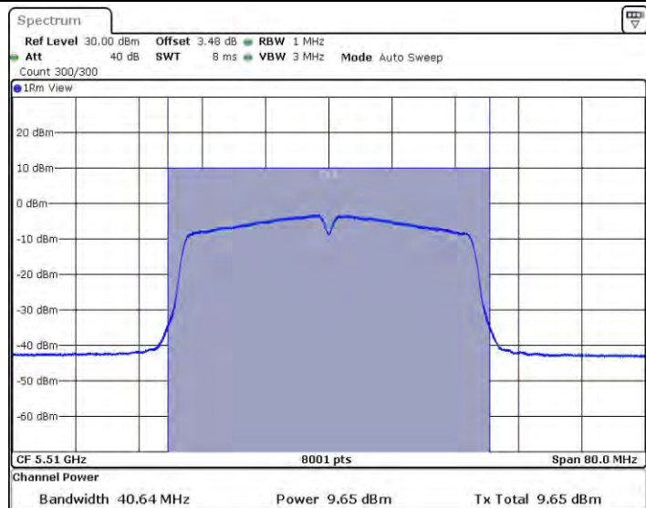
11N40MIMO_Ant2_5510
