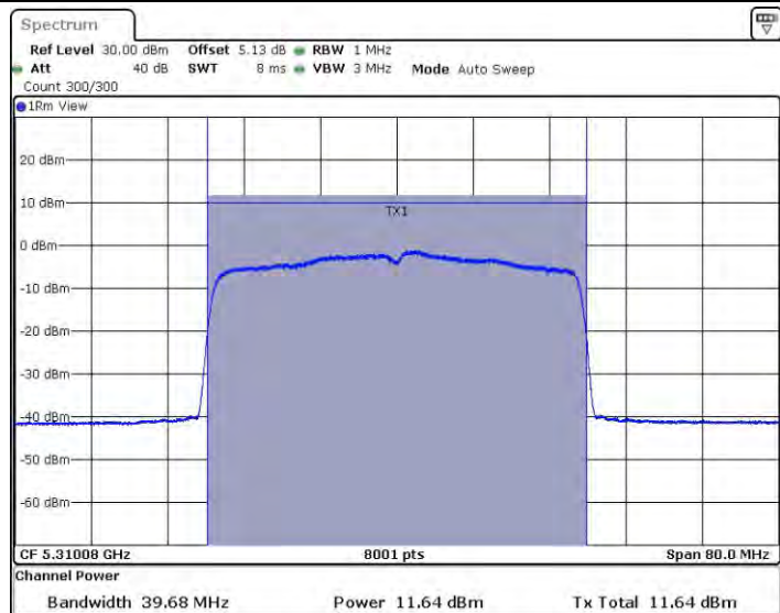
11AX40SISO_Ant2_5310
