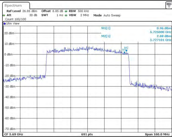
11AX80SISO_Ant1_5690_UNII-3
