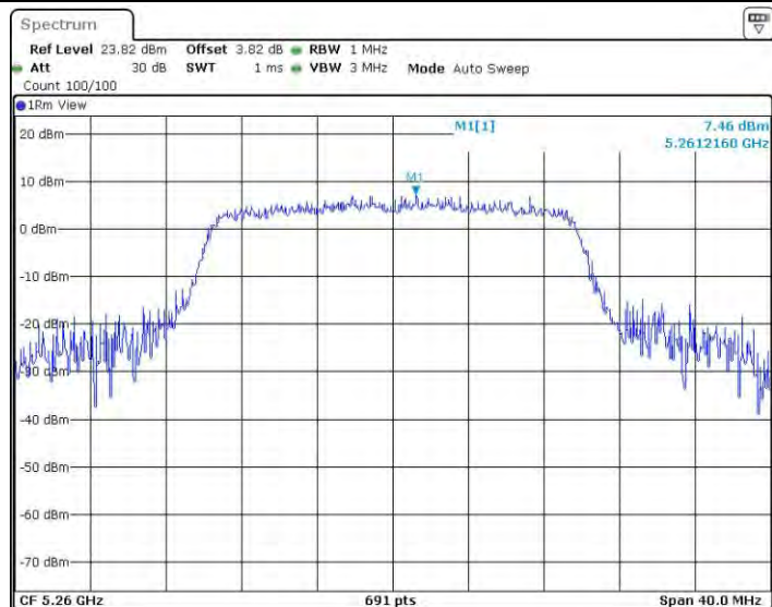
11AX20MIMO_Ant2_5260
