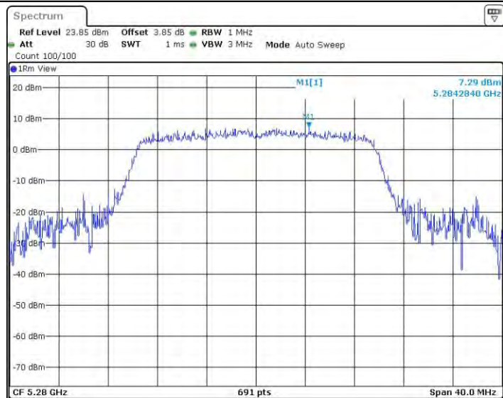
11AX20MIMO_Ant2_5280
