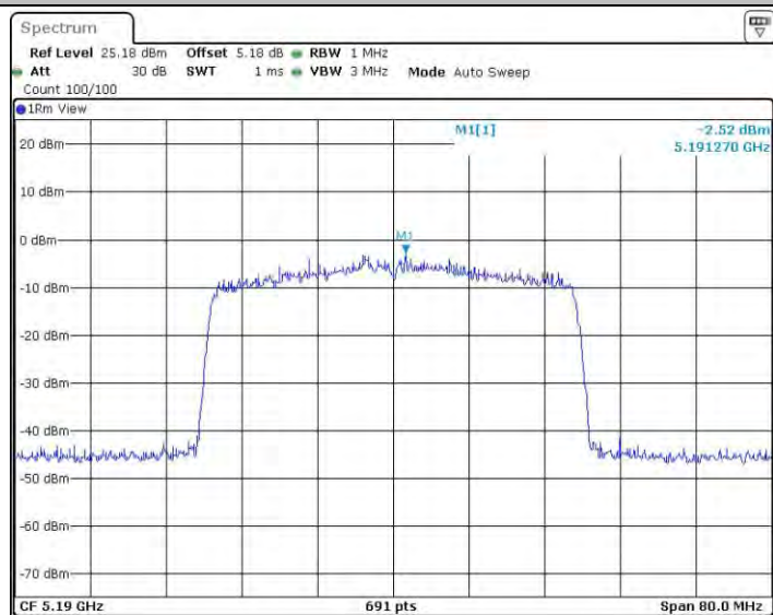
11AX40MIMO_Ant1_5190
