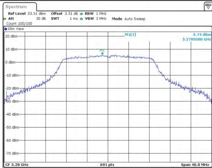
11AC20MIMO_Ant2_5280
