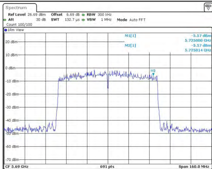
11AC80MIMO_Ant2_5690_UNII-3
