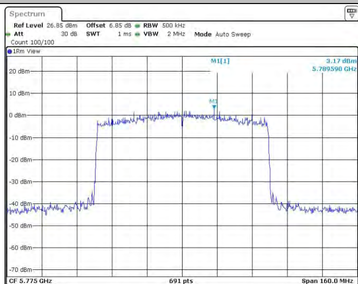
11AX80MIMO_Ant1_5775
