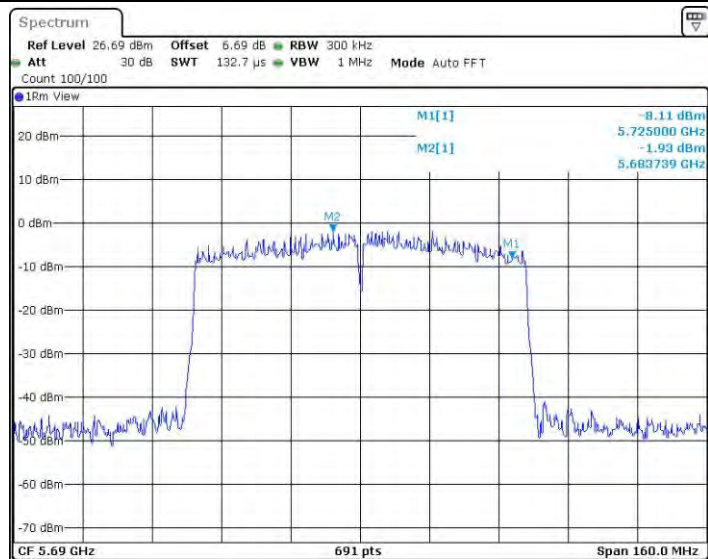
11AC80MIMO_Ant2_5690_UNII-2C
