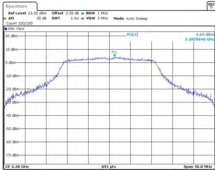
11AC20MIMO_Ant1_5580
