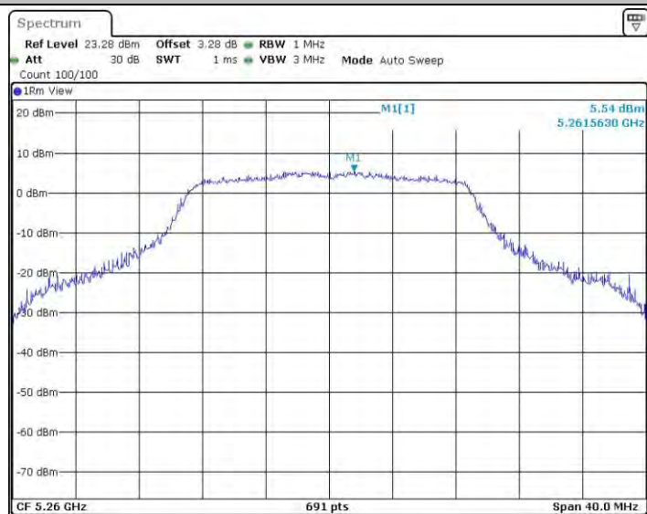
11AC20MIMO_Ant2_5260
