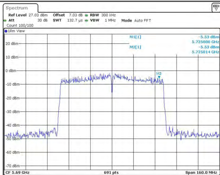
11AC80MIMO_Ant1_5690_UNII-3
