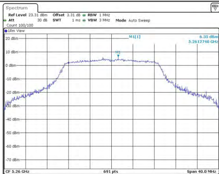
11AC20MIMO_Ant1_5260
