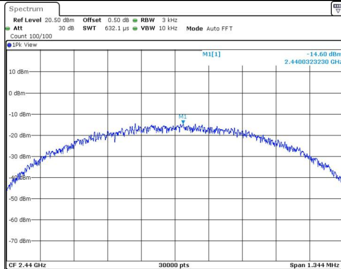
BLE_1M_2440
