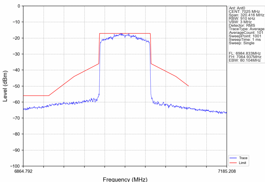
802.11ax(HEW80)_LCH_7025MHz_RU996 / Ant0_NTNV
