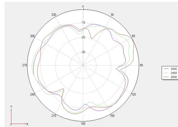
Theta 90 2D图
