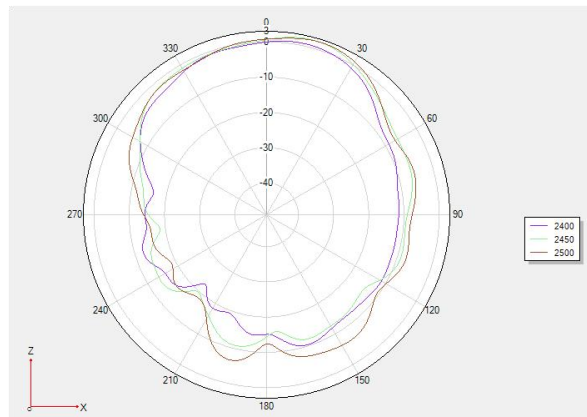
Phi 0 2D图
