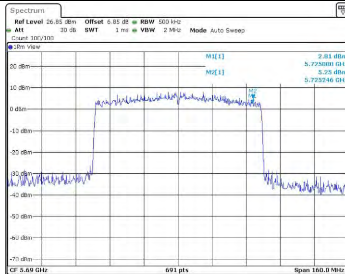
11AX80SISO_Ant1_5690_UNII-3
