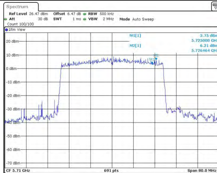
11AX40SISO_Ant2_5710_UNII-3
