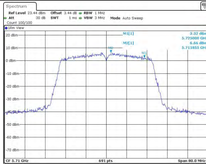
11N40MIMO_Ant2_5710_UNII-2C
