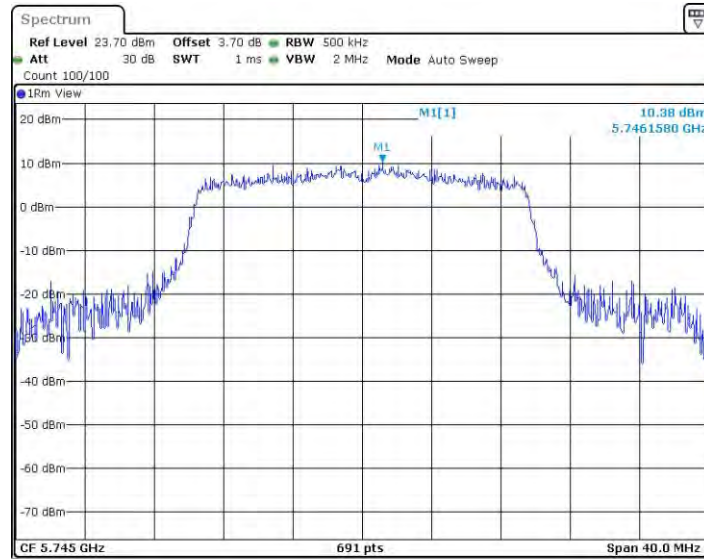
11AX20SISO_Ant2_5745
