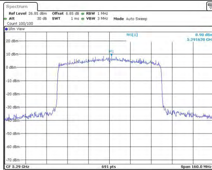
11AX80SISO_Ant2_5290
