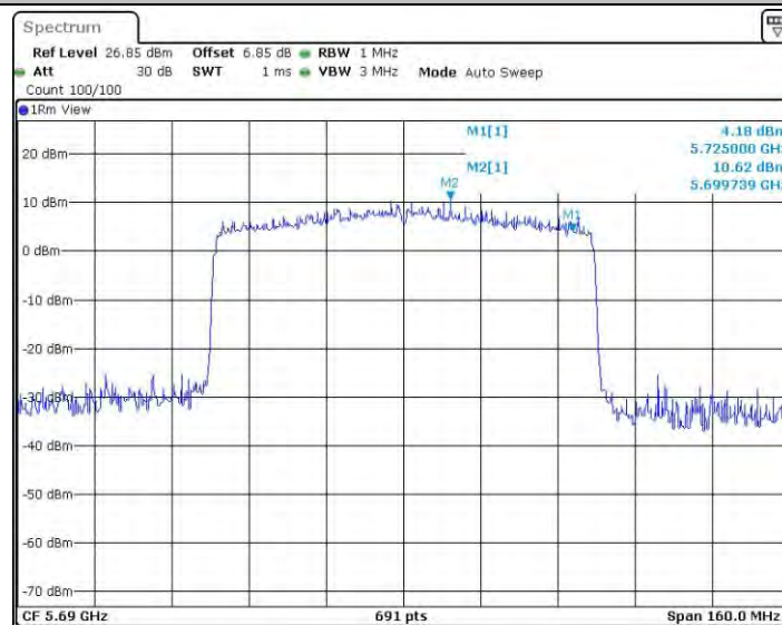
11AX80SISO_Ant1_5690_UNII-2C
