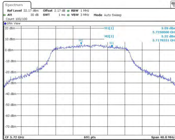
11N20MIMO_Ant2_5720_UNII-2C
