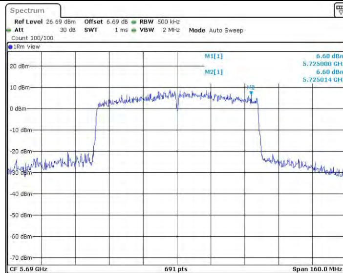
11AC80SISO_Ant2_5690_UNII-3
