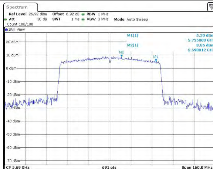
11AC80SISO_Ant1_5690_UNII-2C
