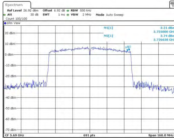
11AC80SISO_Ant1_5690_UNII-3
