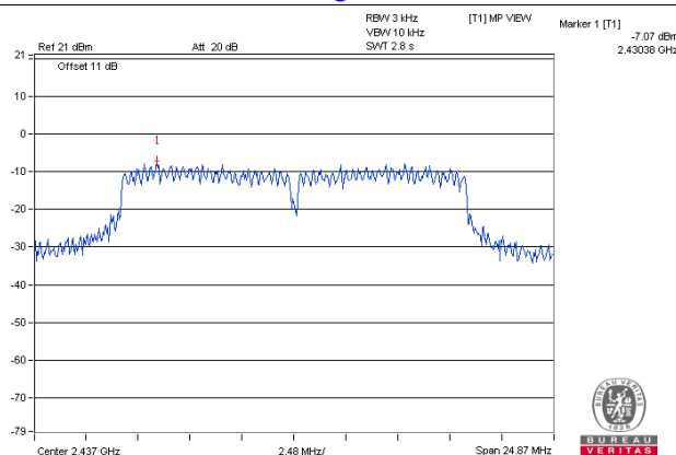
802.11g : CH6
