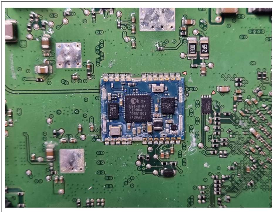
< GPS Module>
