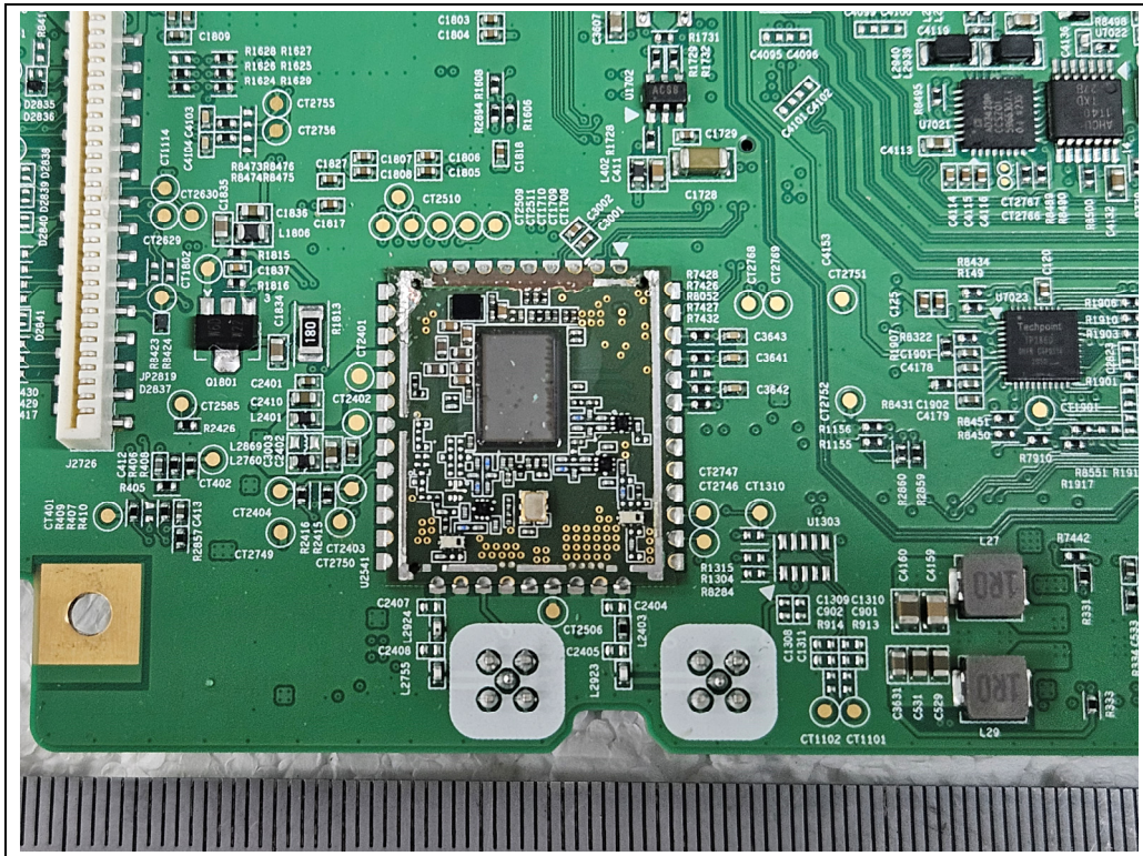
<BT/WLAN Module>
