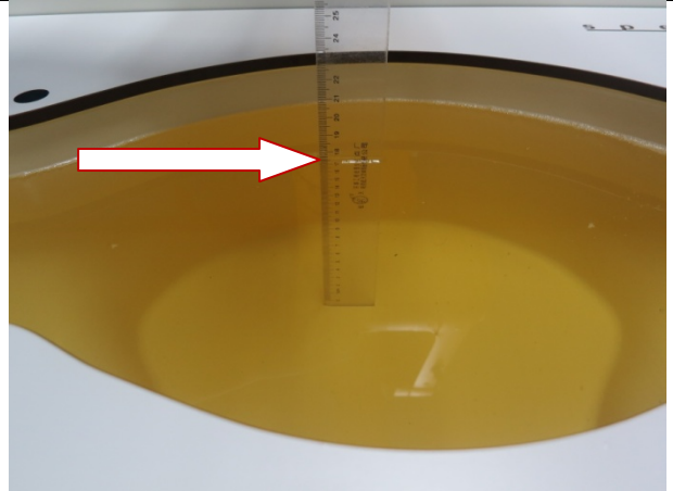
2450MHz body
