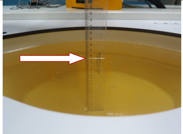
1900MHz body
