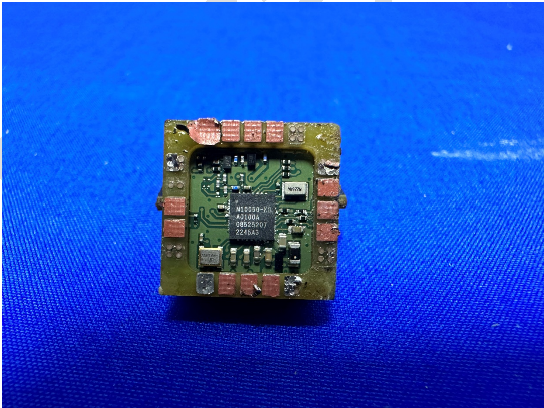
(14) EUT Photo
