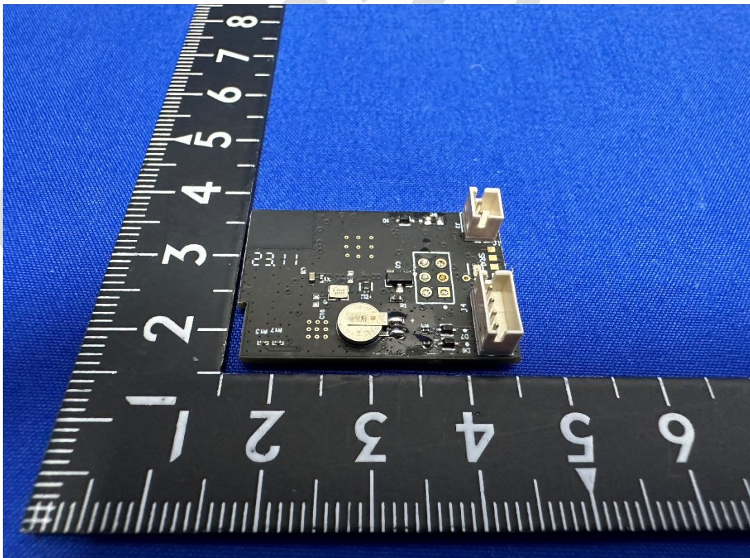
(10) EUT Photo
