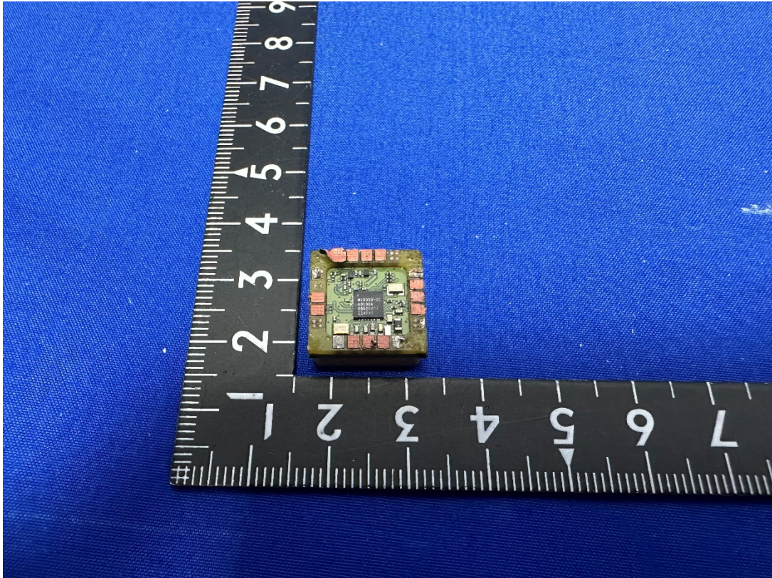
(14) EUT Photo
