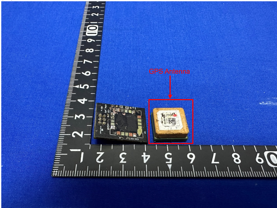
(12) EUT Photo
