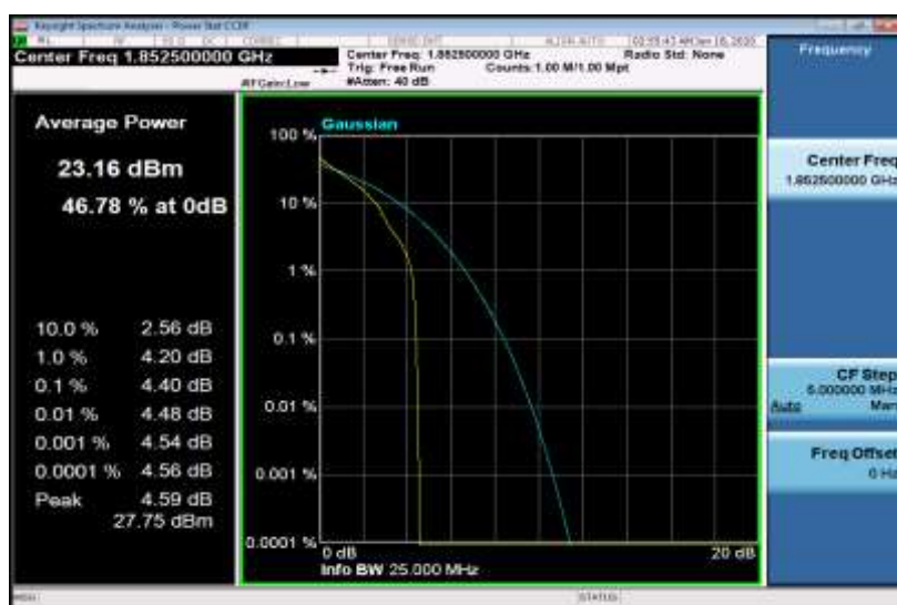
Band2-5MHz-QPSK-18625-25RB#0
