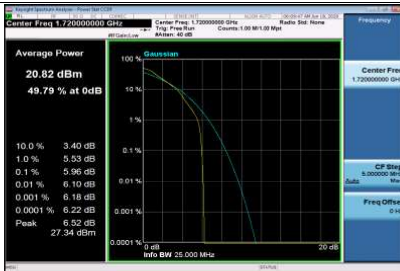
Band4-20MHz-QPSK-20050-100RB#0
