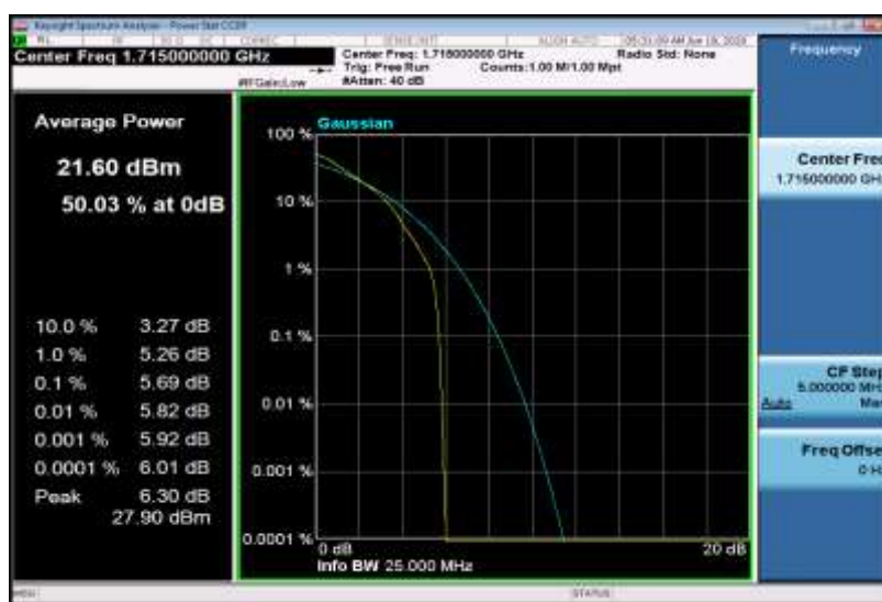
Band4-10MHz-QPSK-20000-50RB#0
