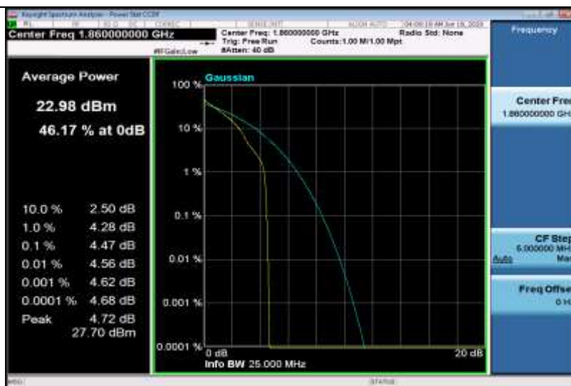
Band2-20MHz-QPSK-18700-100RB#0
