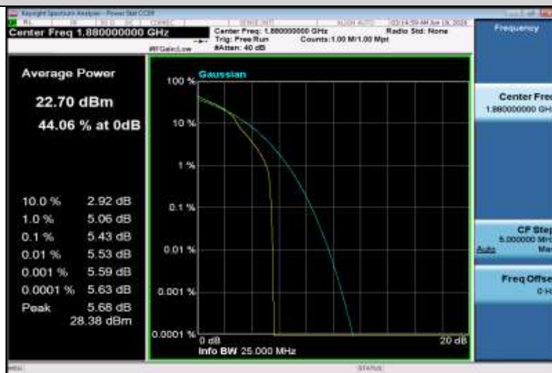
Band2-10MHz-16QAM-18900-50RB#0
