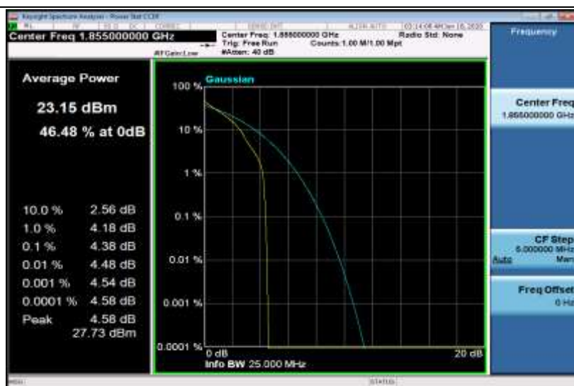
Band2-10MHz-QPSK-18650-50RB#0
