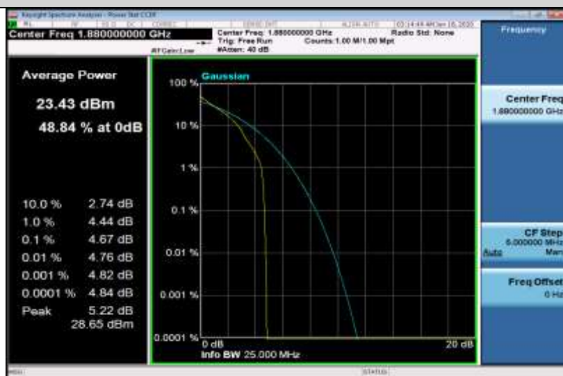
Band2-10MHz-QPSK-18900-50RB#0
