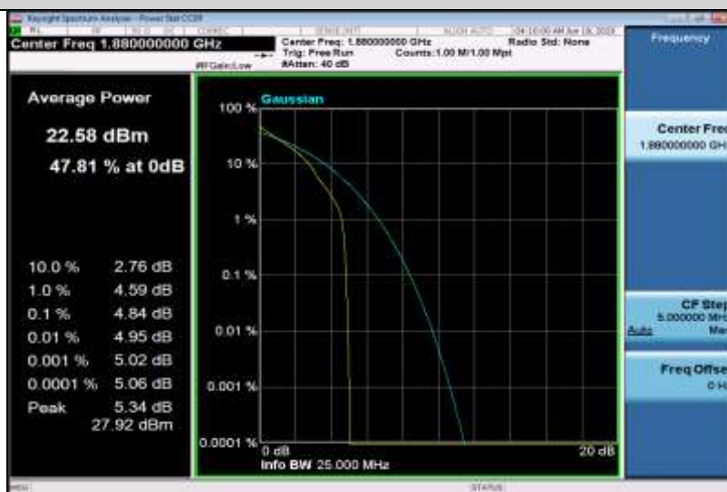
Band2-20MHz-QPSK-18900-100RB#0
