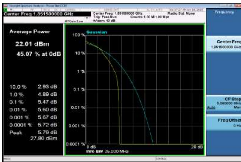
Band2-3MHz-16QAM-18615-15RB#0
