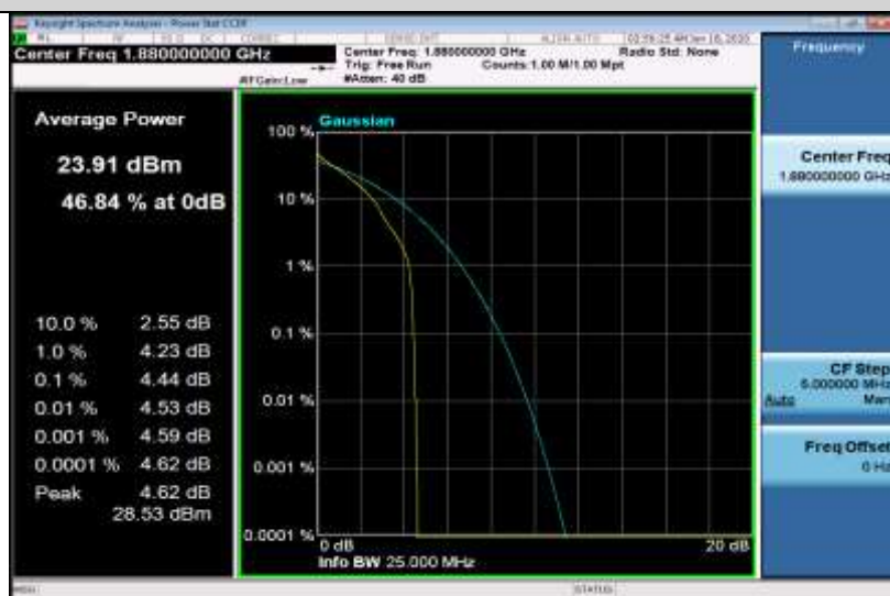
Band2-5MHz-QPSK-18900-25RB#0
