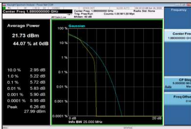
Band2-20MHz-16QAM-18900-100RB#0
