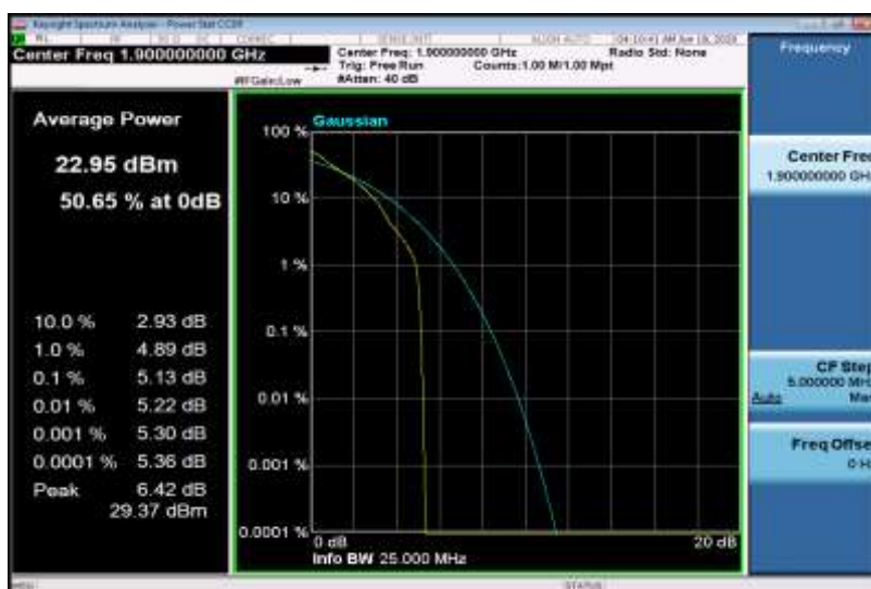
Band2-20MHz-QPSK-19100-100RB#0
