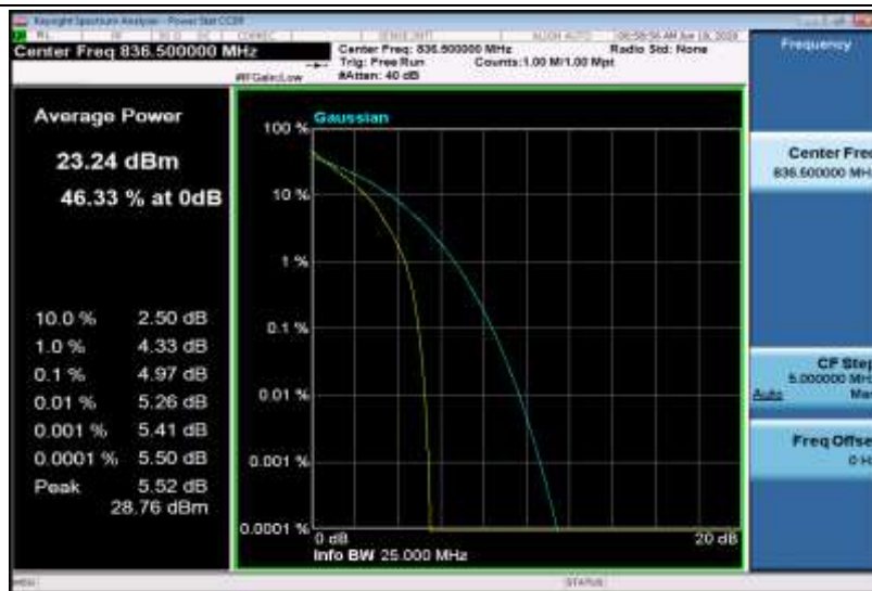
Band5-3MHz-QPSK-20635-1RB#0
