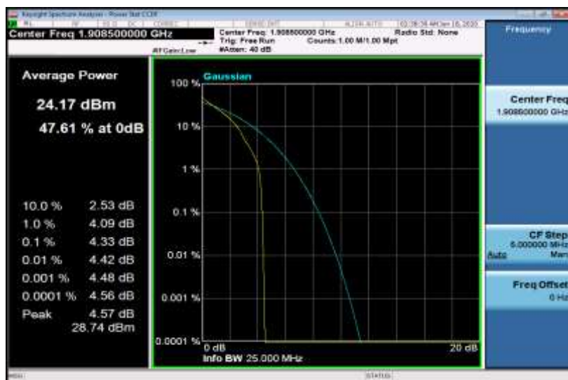
Band2-3MHz-QPSK-19185-15RB#0
