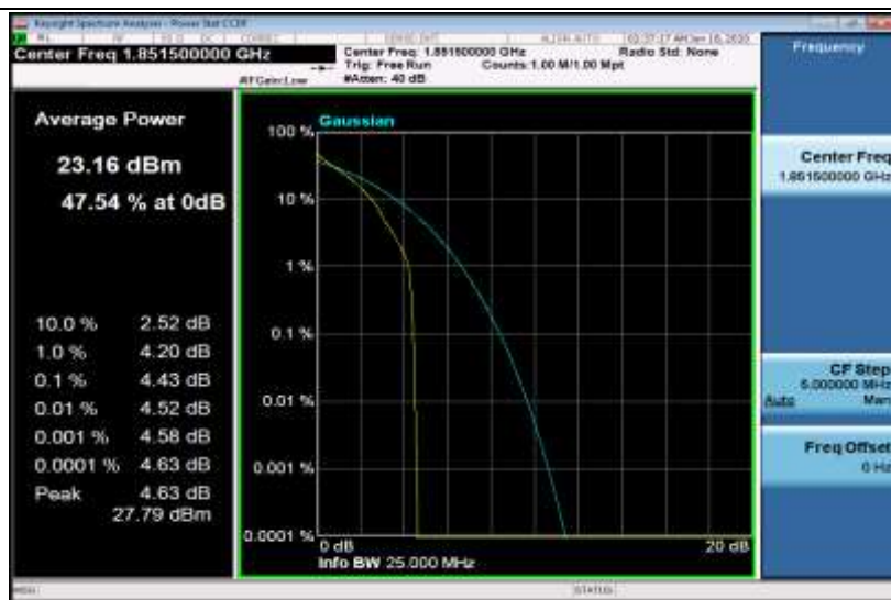
Band2-3MHz-QPSK-18615-15RB#0
