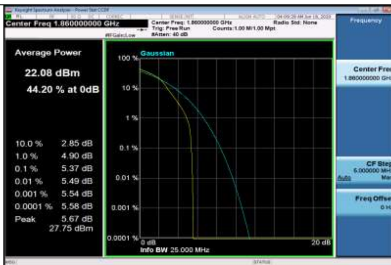
Band2-20MHz-16QAM-18700-100RB#0
