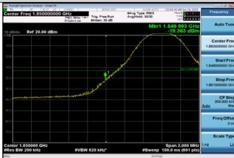
Band2-10MHz-QPSK-18650-1RB#0
