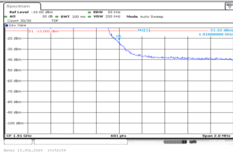
Band2-3MHz-QPSK-19185-15RB#0
