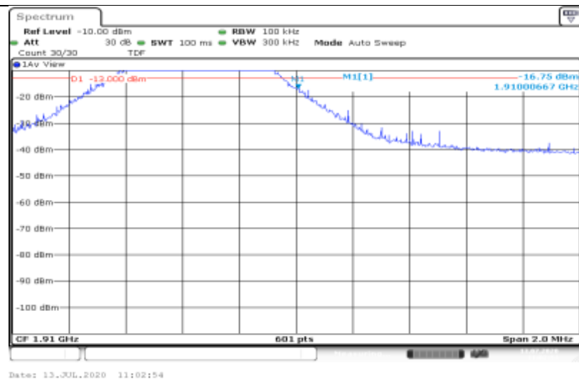
Band2-5MHz-QPSK-19175-1RB#0
