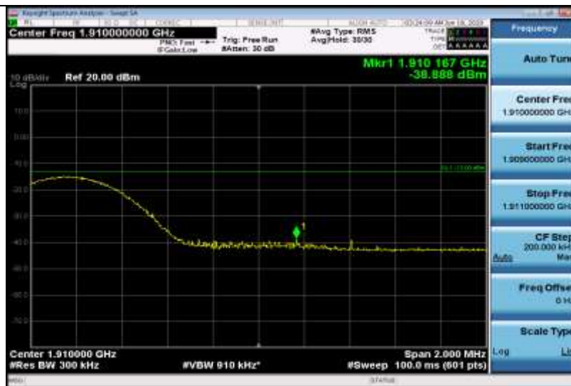
Band2-15MHz-16QAM-19125-1RB#74
