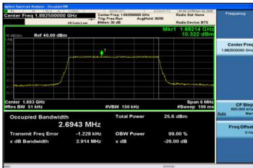
Band25-3MHz-QPSK-26675-15RB#0-2.6965
