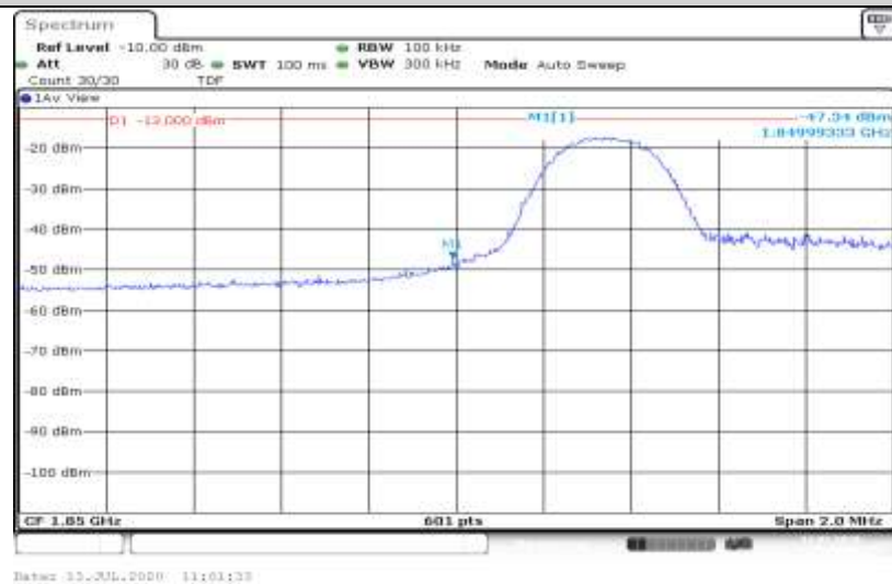
Band2-5MHz-QPSK-18625-1RB#24
