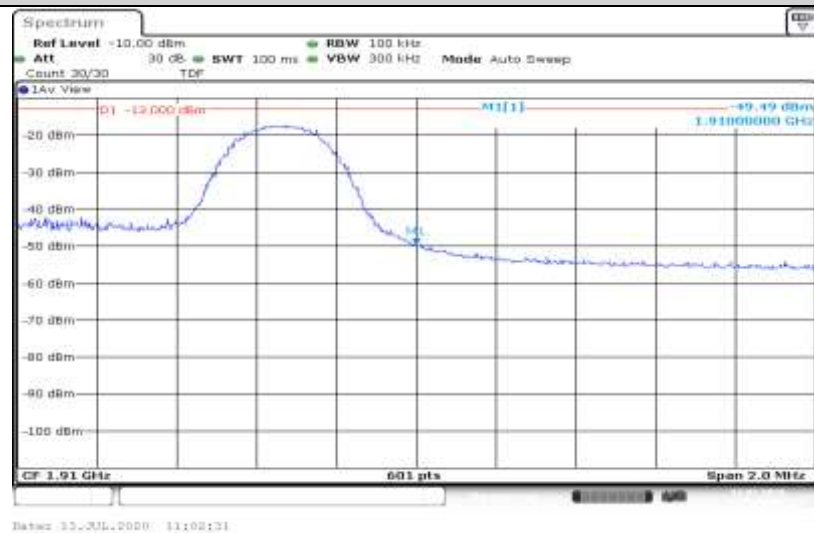
Band2-5MHz-QPSK-19175-1RB#0
