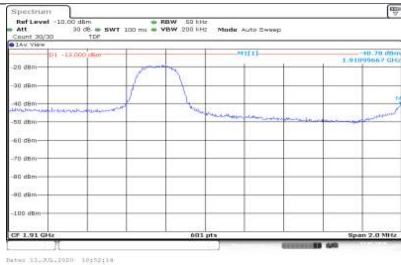
Band2-3MHz-QPSK-19185-1RB#14
