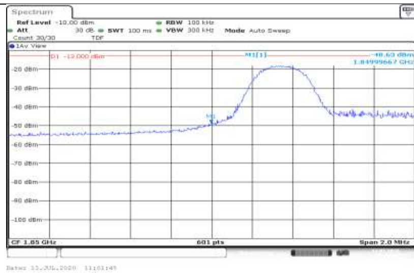
Band2-5MHz-16QAM-18625-1RB#0
