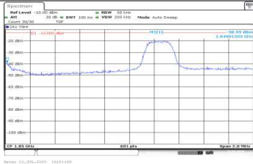
Band2-3MHz-16QAM-18615-15RB#0
