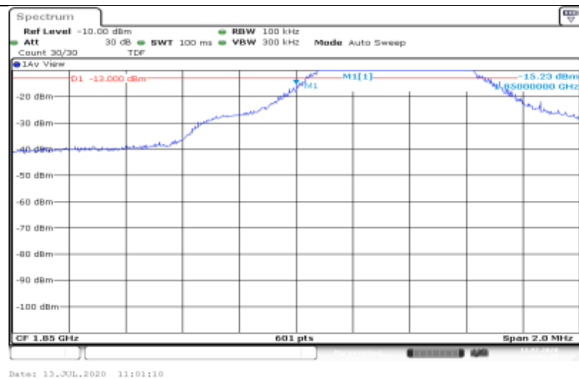
Band2-5MHz-QPSK-18625-1RB#24
