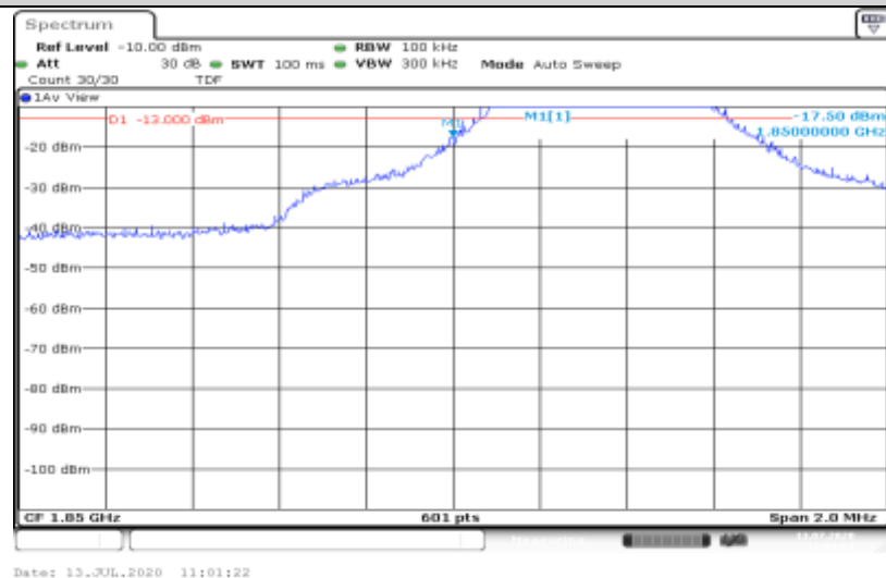
Band2-5MHz-16QAM-18625-1RB#0
