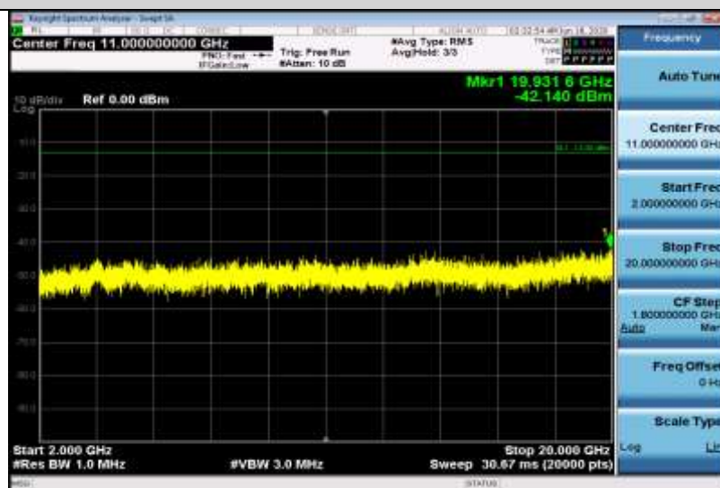
Band2-3MHz-QPSK-19185-1RB#0-Range3:2000~20000MHz
