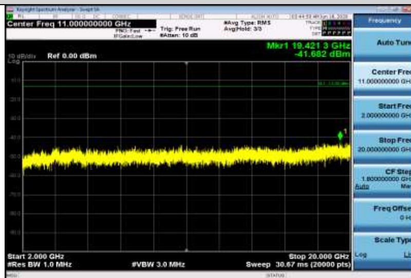
Band2-20MHz-QPSK-18700-1RB#0-Range3:2000~20000MHz
