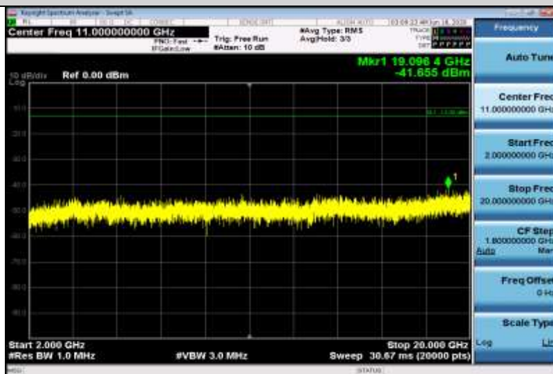
Band2-10MHz-QPSK-19150-1RB#0-Range3:2000~20000MHz
