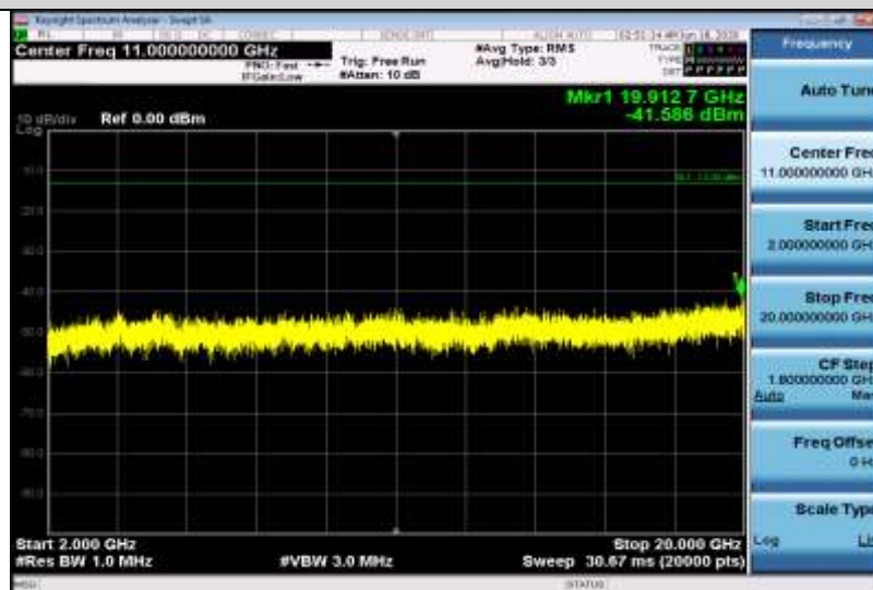
Band2-5MHz-QPSK-19175-1RB#0-Range3:2000~20000MHz
