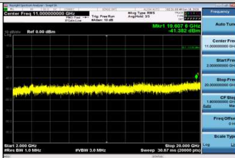
Band2-3MHz-QPSK-18615-1RB#0-Range3:2000~20000MHz
