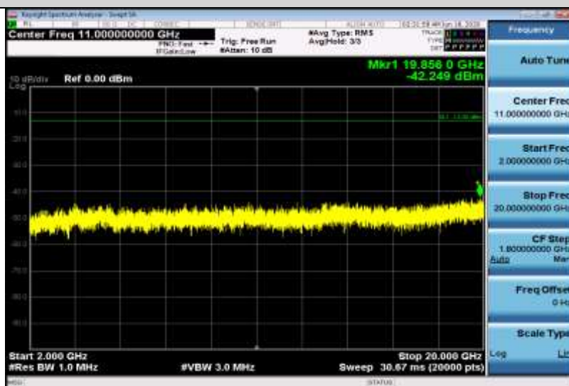
Band2-3MHz-QPSK-18900-1RB#0-Range3:2000~20000MHz
