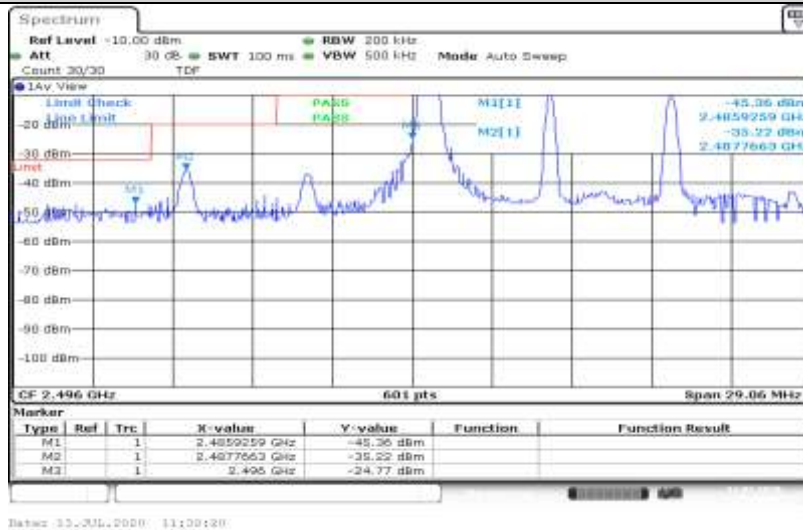
Band41-10MHz-QPSK-39700-50RB#0
