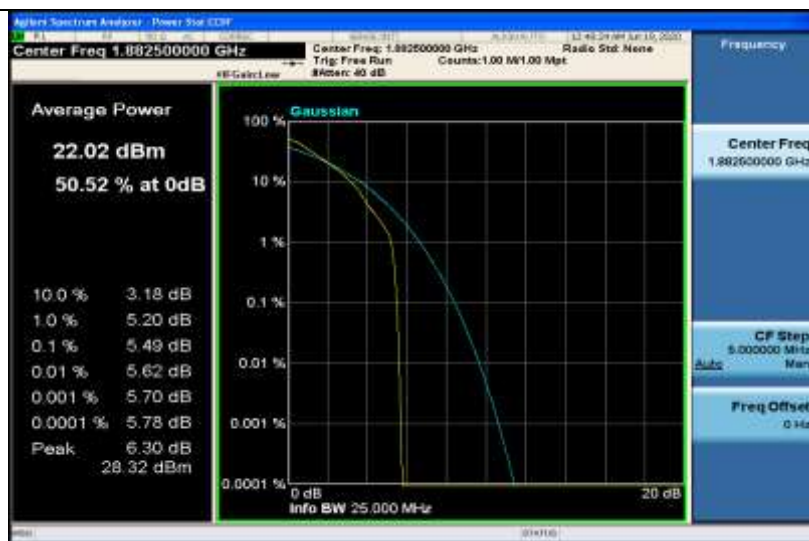
Band25-20MHz-QPSK-26365-100RB#0
