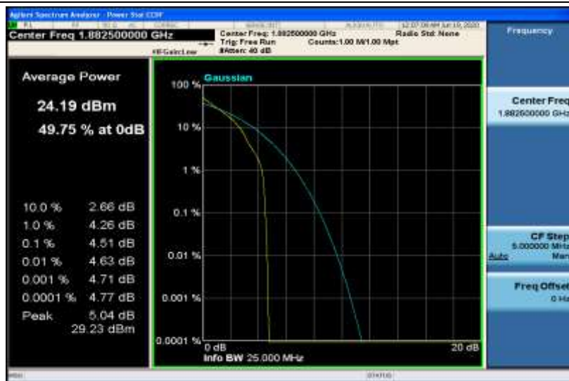
Band25-10MHz-QPSK-26365-50RB#0
