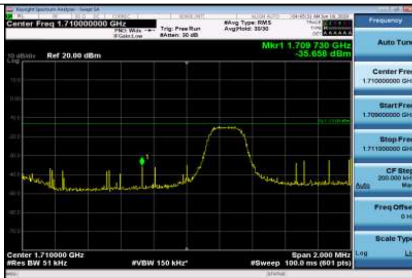
Band4-3MHz-QPSK-19965-1RB#0
