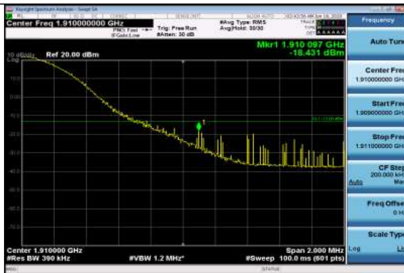
Band2-20MHz-16QAM-19100-1RB#0
