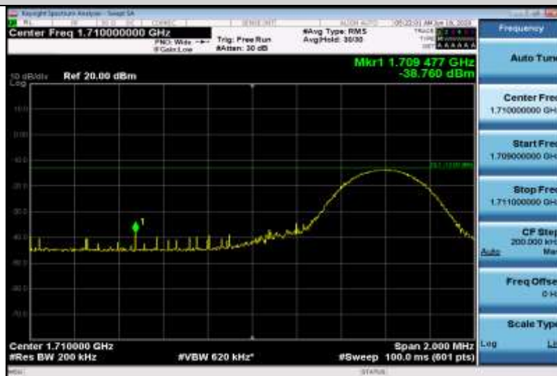
Band4-10MHz-QPSK-20000-50RB#0
