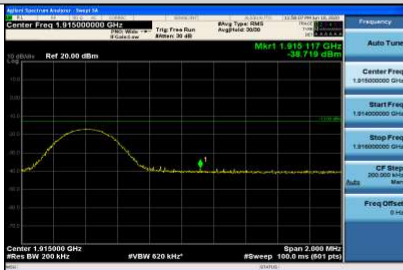
Band25-10MHz-QPSK-26640-50RB#0
