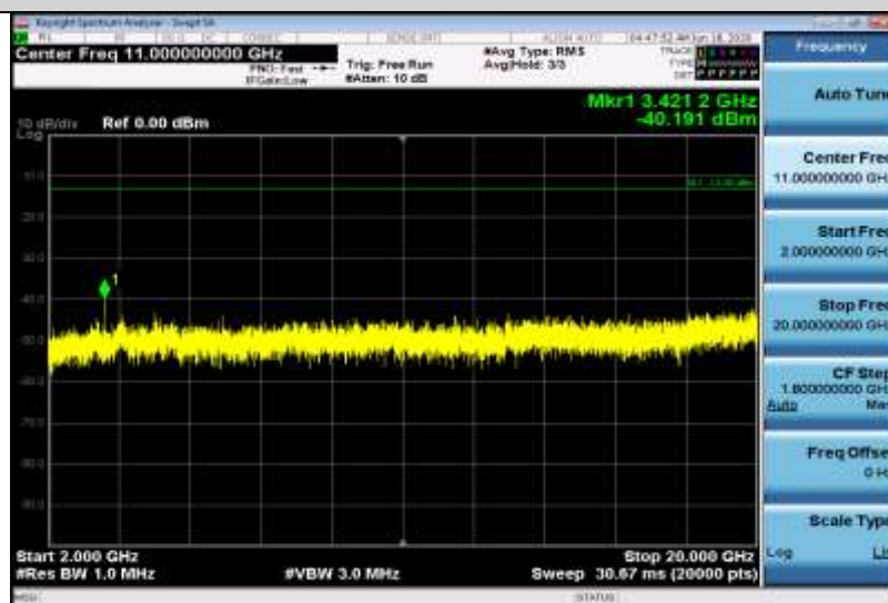
Band4-3MHz-QPSK-19965-1RB#0-Range3:2000~20000MHz
