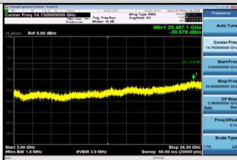
Band7-20MHz-QPSK-21350-1RB#0-Range3:3000~26500MHz
