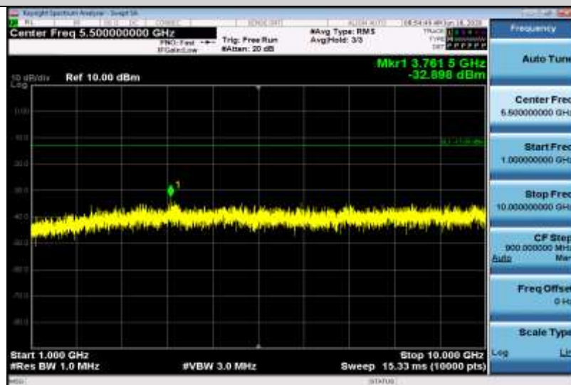
Band12-5MHz-QPSK-23155-1RB#0-Range2:1000~10000MHz
