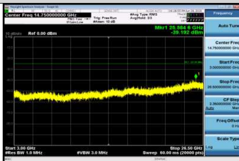
Band7-5MHz-QPSK-21425-1RB#0-Range3:3000~26500MHz
