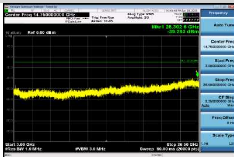
Band7-20MHz-QPSK-21100-1RB#0-Range3:3000~26500MHz
