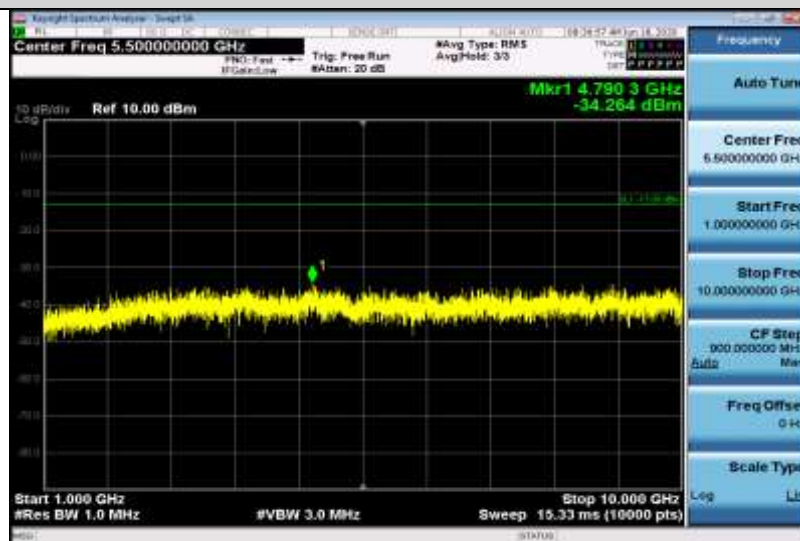
Band12-3MHz-QPSK-23165-1RB#0-Range2:1000~10000MHz
