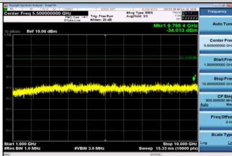
Band5-3MHz-QPSK-20635-1RB#0-Range2:1000~10000MHz
