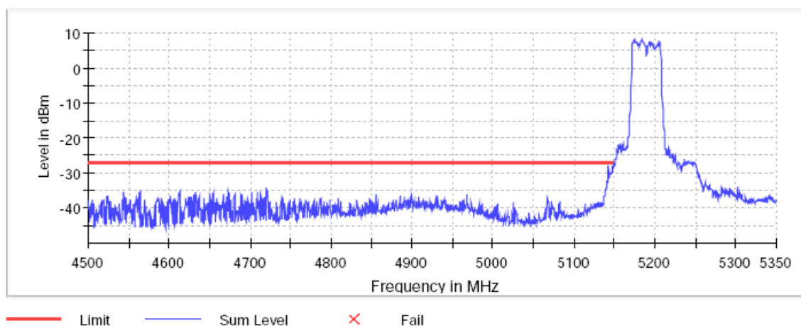
Band Edge
