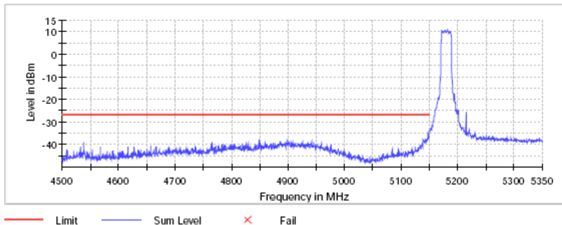
Band Edge
