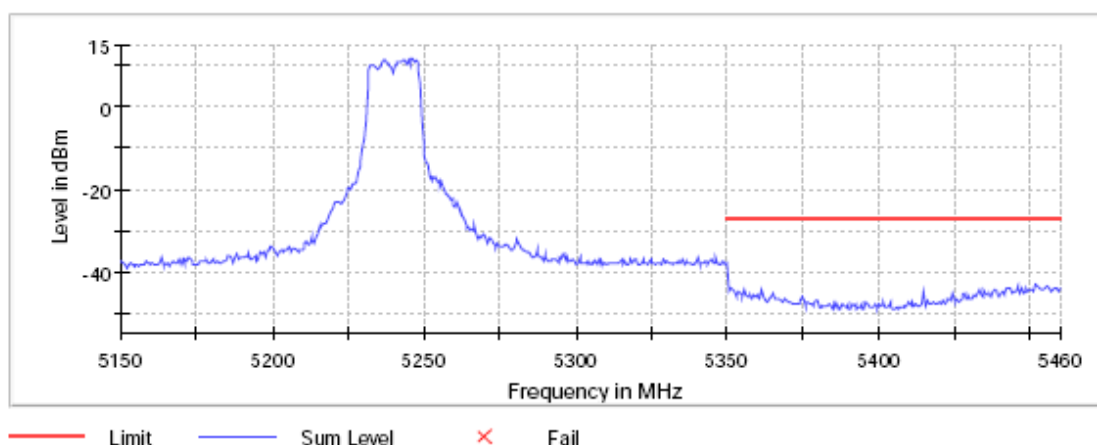
Band Edge
