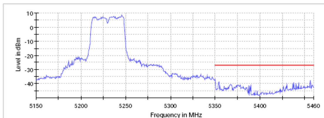
Band Edge
