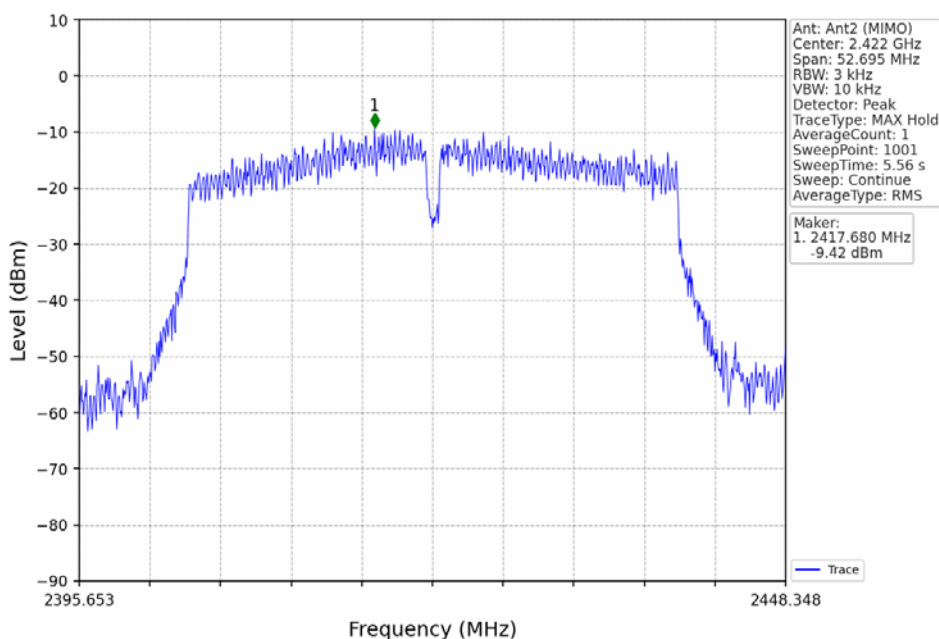
802.11n(HT40)_LCH_2422MHz_MIMO_NTNV
