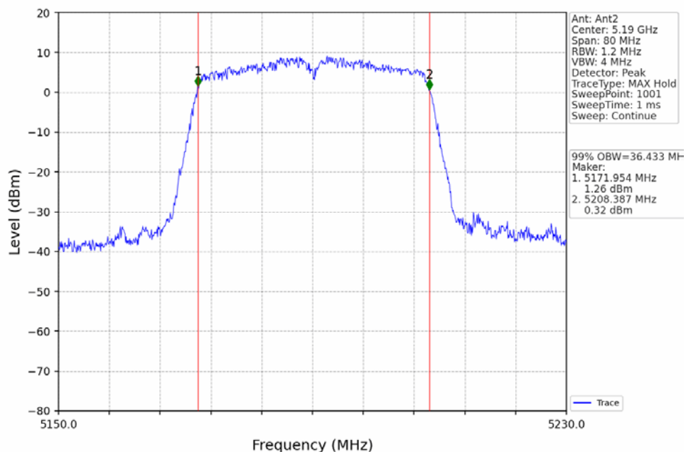
802.11n(HT40)_LCH_5190MHz_Ant2_NTNV
