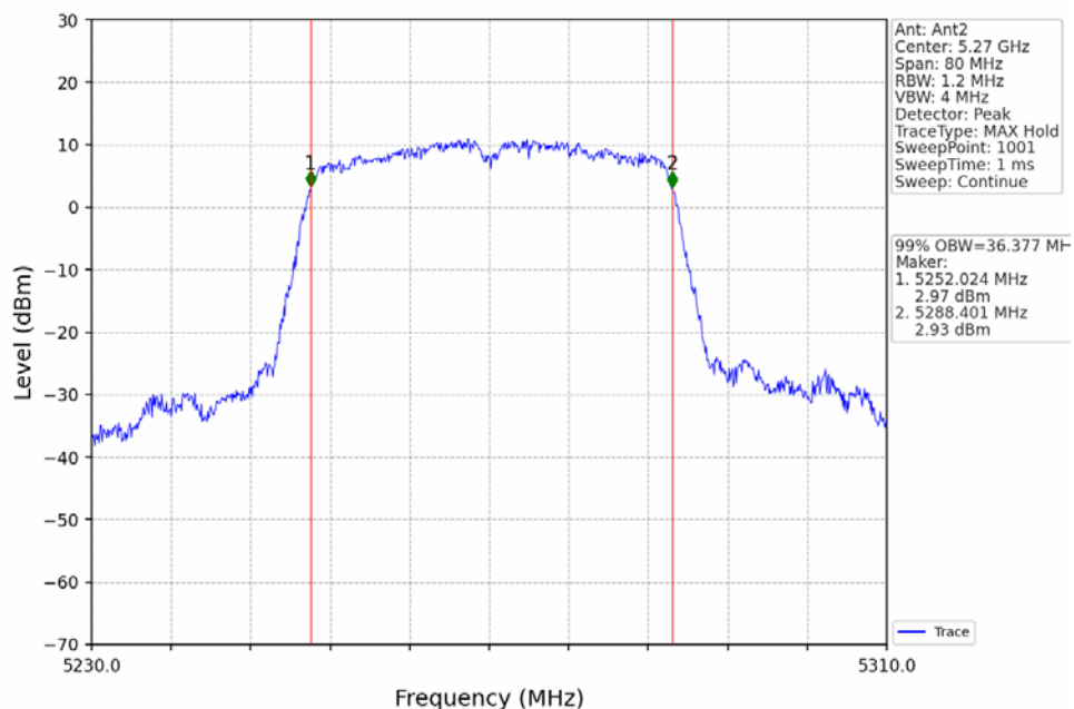
802.11n(HT40)_LCH_5270MHz_Ant2_NTNV
