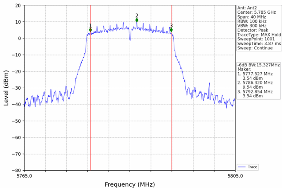
802.11a_MCH_5785MHz_Ant2_NTNV
