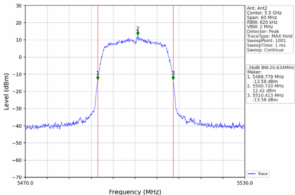
802.11n(HT20)_LCH_5500MHz_Ant2_NTNV
