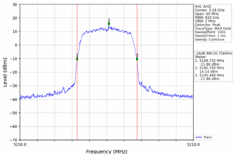
802.11n(HT20)_LCH_5180MHz_Ant2_NTNV
