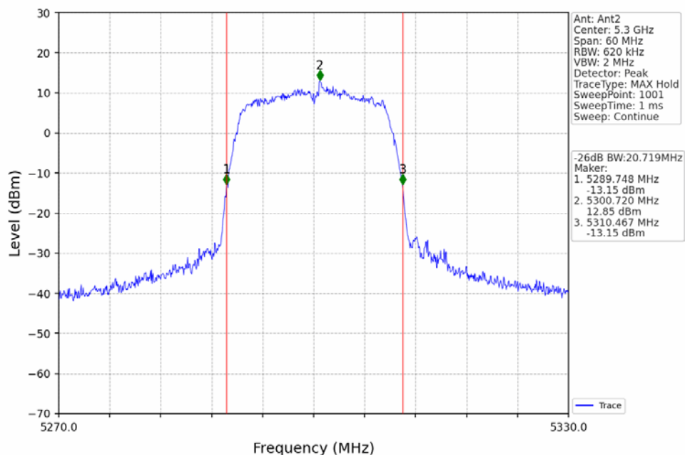
802.11n(HT20)_MCH_5300MHz_Ant2_NTNV
