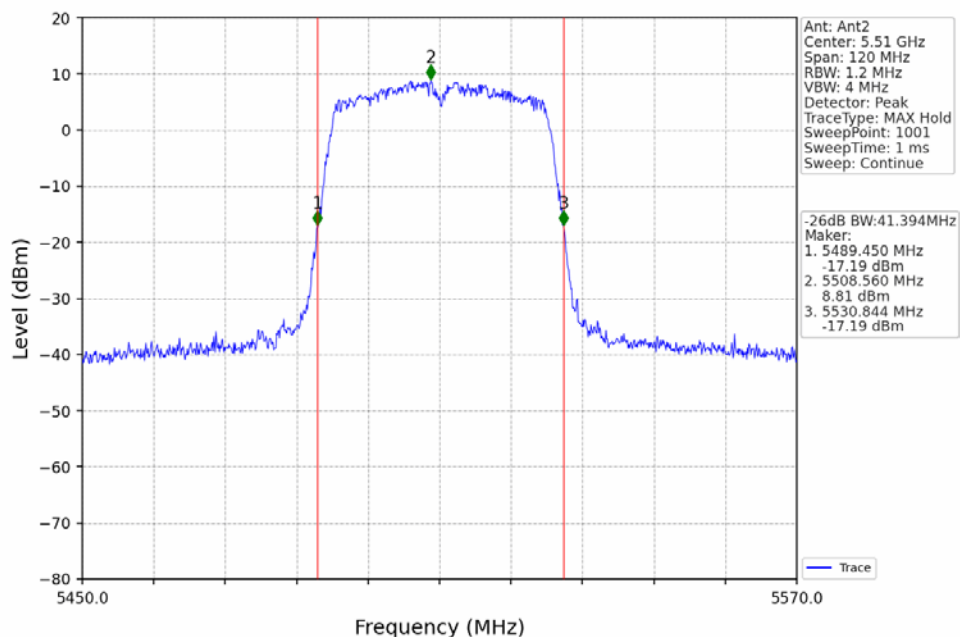
802.11n(HT40)_LCH_5510MHz_Ant2_NTNV
