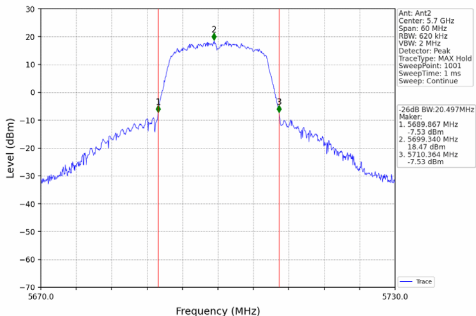
802.11a_HCH_5700MHz_Ant2_NTNV
