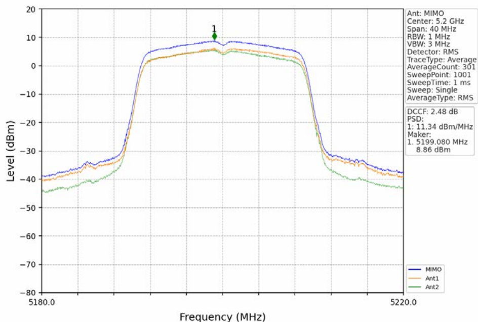
802.11n(HT20)_MCH_5200MHz_MIMO_NTNV
