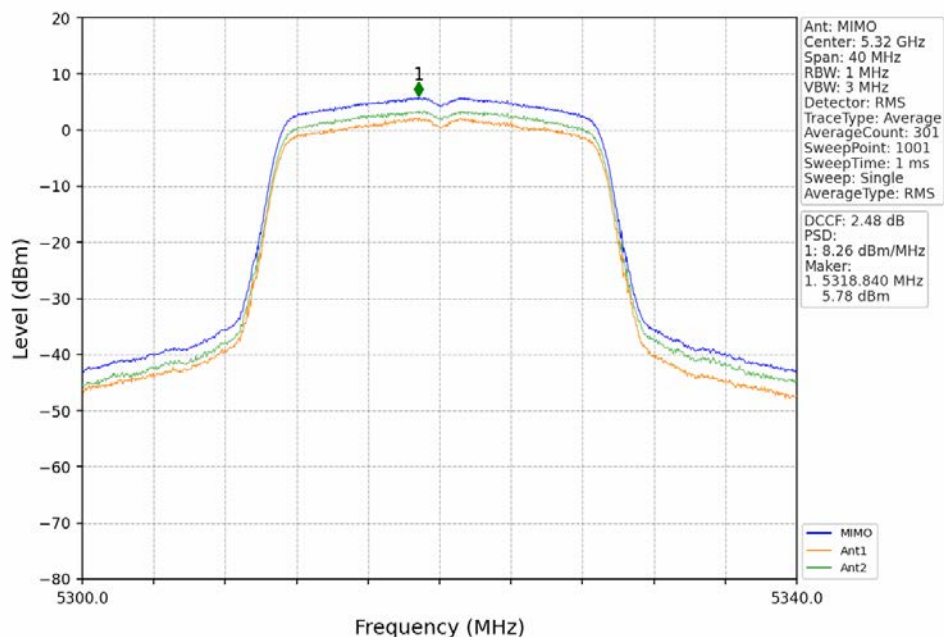
802.11n(HT20)_HCH_5320MHz_MIMO_NTNV
