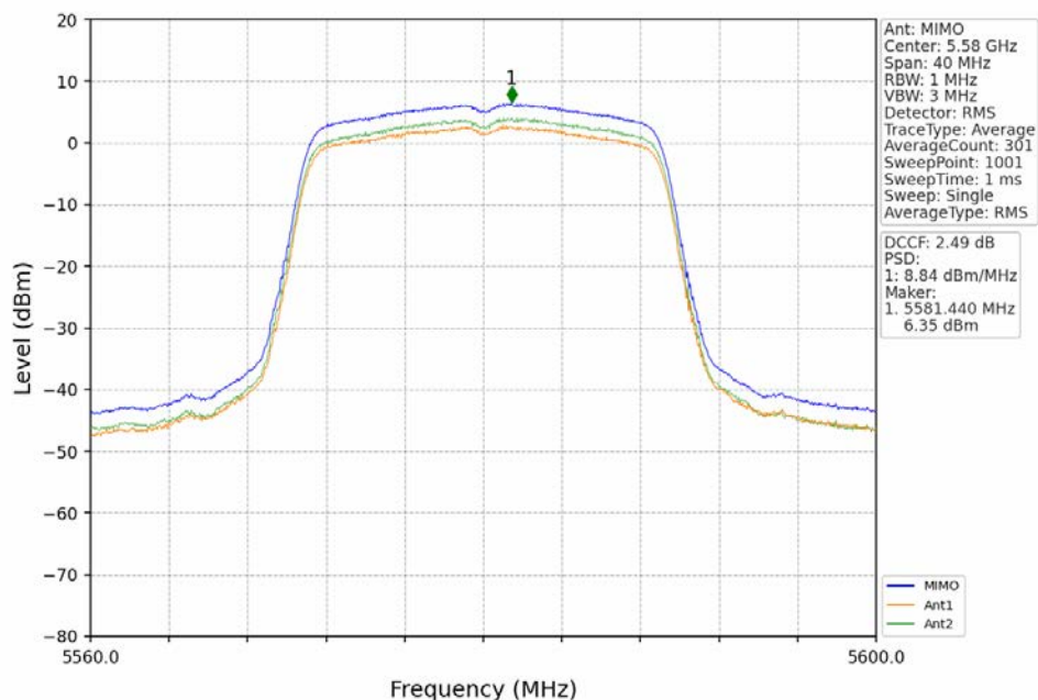
802.11n(HT20)_MCH_5580MHz_MIMO_NTNV
