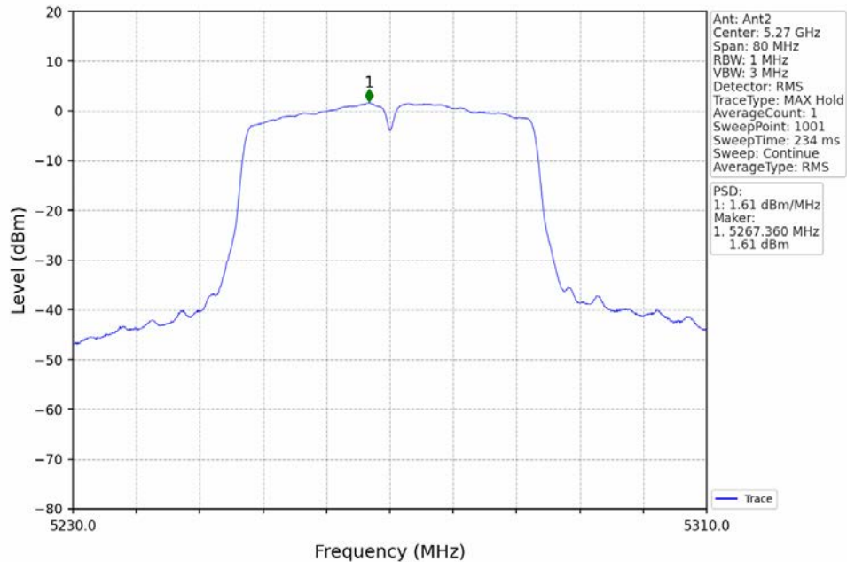
802.11n(HT40)_LCH_5270MHz_MIMO_NTNV
