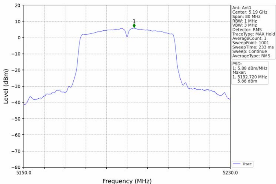
802.11n(HT40)_LCH_5190MHz_Ant1_NTNV
