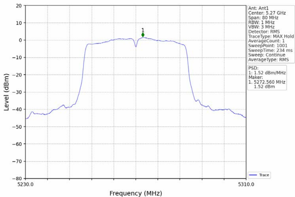
802.11n(HT40)_LCH_5270MHz_Ant1_NTNV
