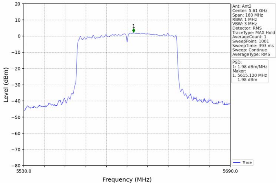
802.11ac(VHT80)_HCH_5610MHz_MIMO_NTNV
