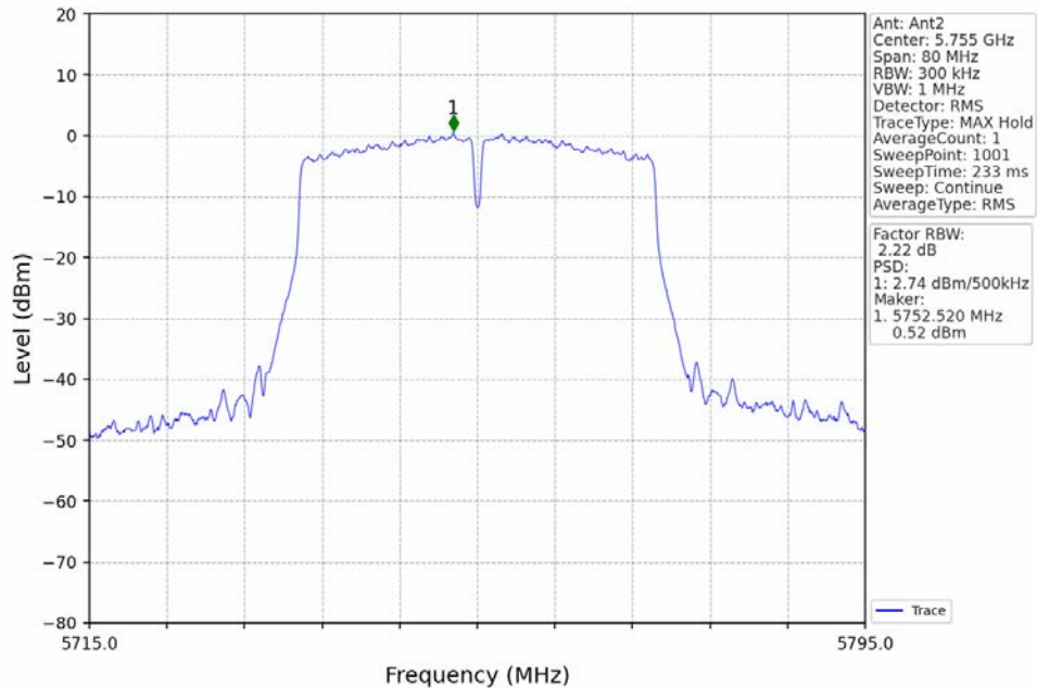
802.11n(HT40)_LCH_5755MHz_MIMO_NTNV
