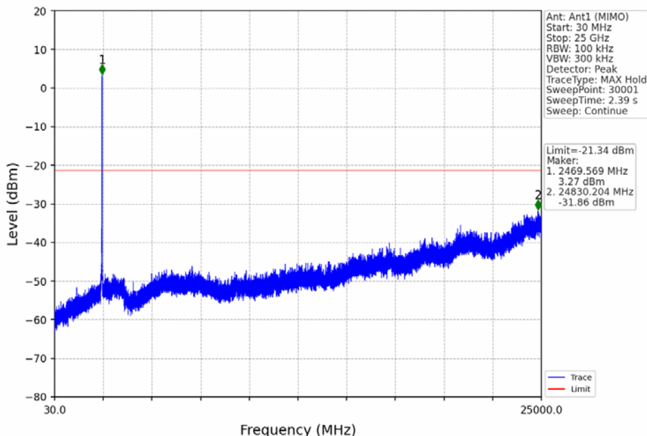
802.11n(HT20)_HCH_2462MHz_Ant1 (MIMO)_NTNV
