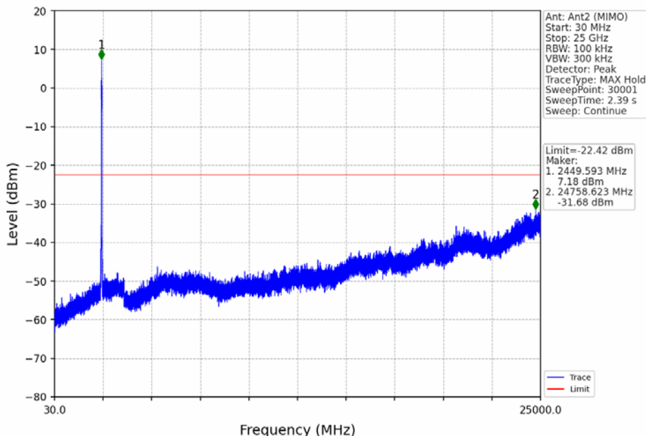
802.11n(HT40)_HCH_2452MHz_Ant2 (MIMO)_NTNV
