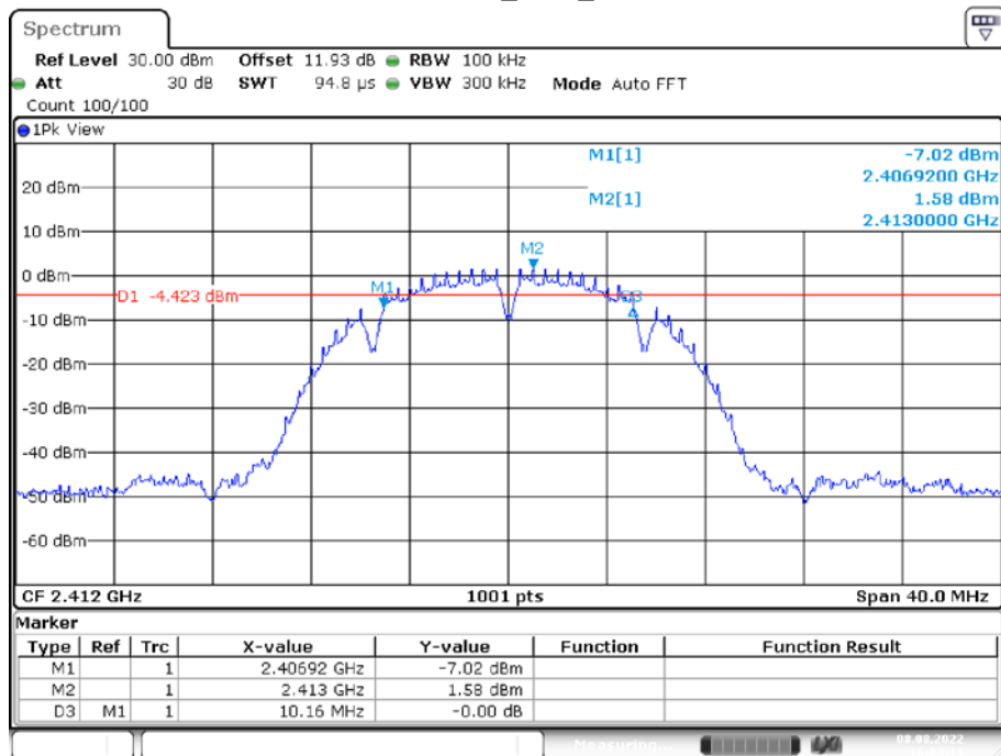
11B MIMO_Ant1_2412
