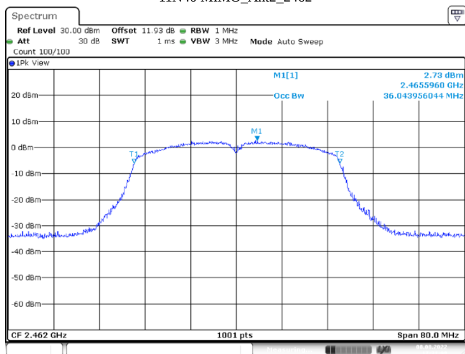
11N40 MIMO_Ant2_2462
