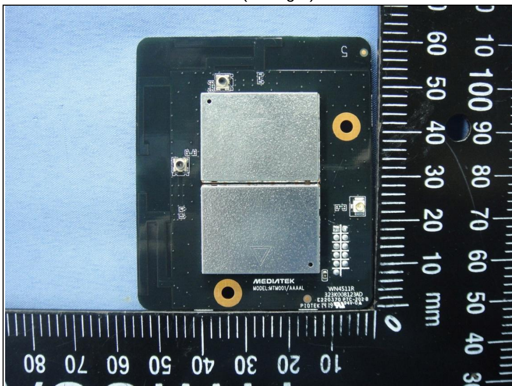
EUT (Config-1)
