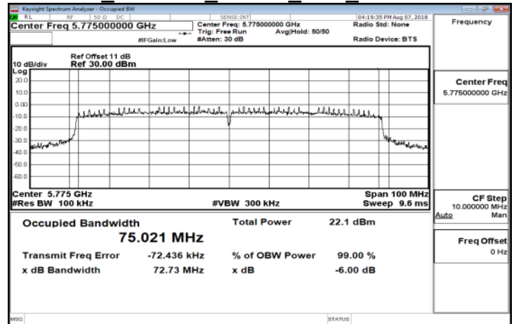
FCC 802.11ac 80MHz CH1 5775MHz
