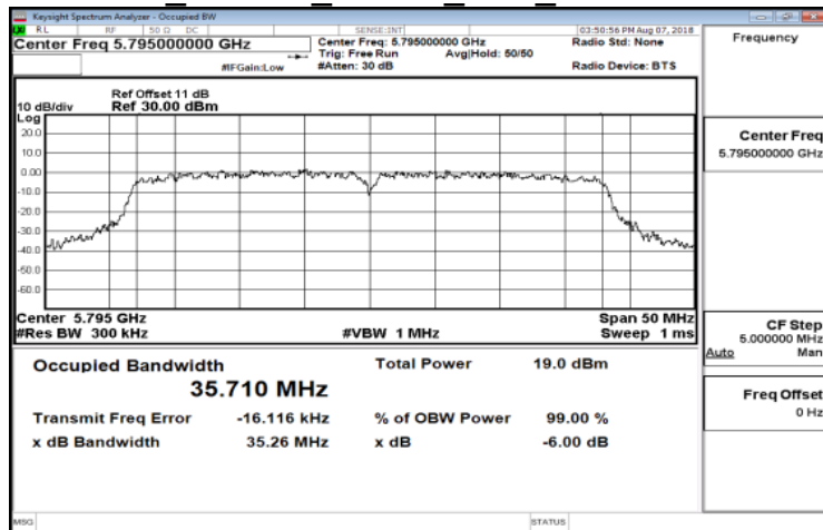
IC 802.11n 40MHz CH1 5795MHz
