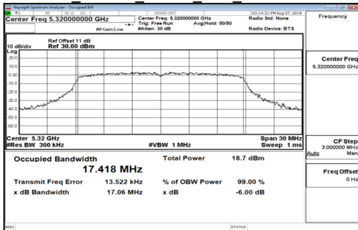
IC 802.11n 20MHz CH1 5320MHz
