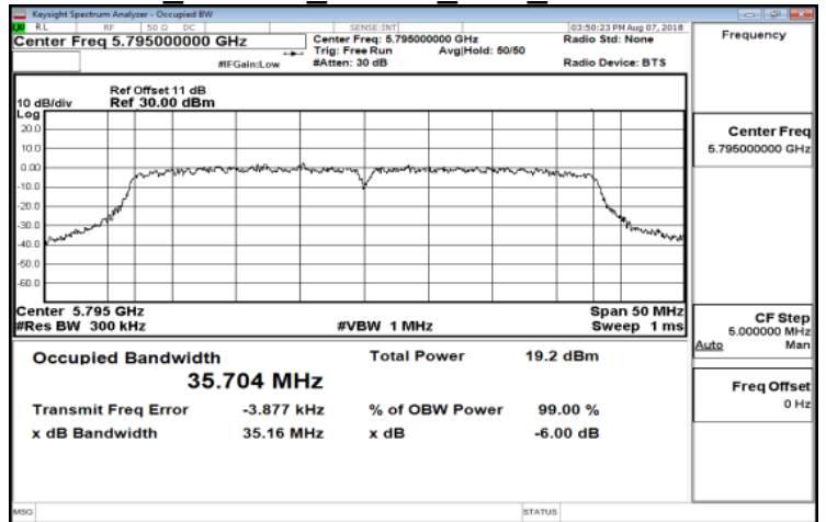
IC 802.11n 40MHz CH0 5795MHz
