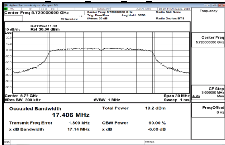
IC 802.11n 20MHz CH0 5720MHz
