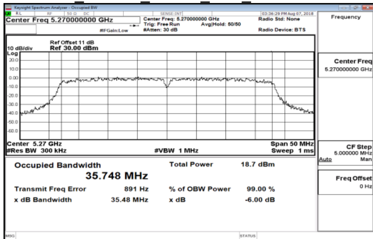
IC 802.11n 40MHz CH0 5270MHz
