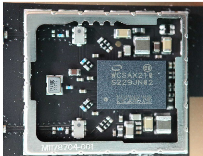
WiFi/BT Module
