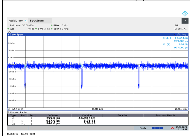
802.11be EHT160 996T+484T (N) MODE
