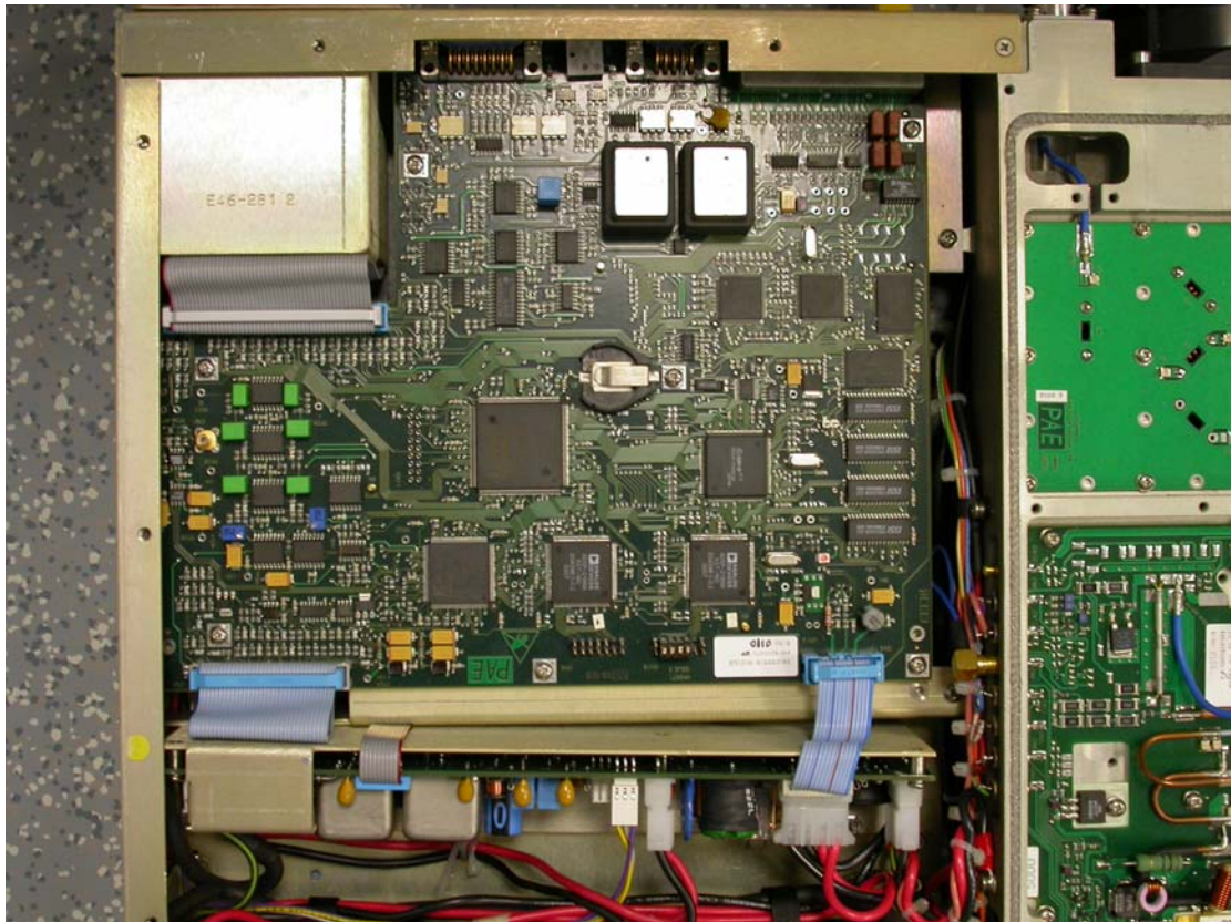
T6T Processor Module
