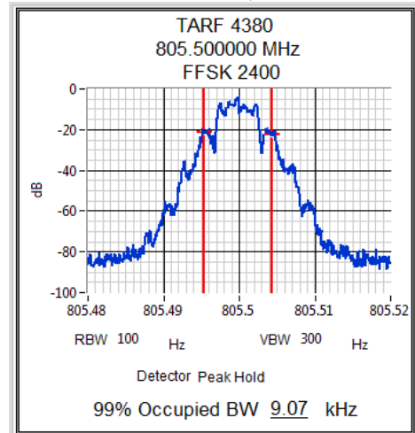
805.500 MHz, 30 W
