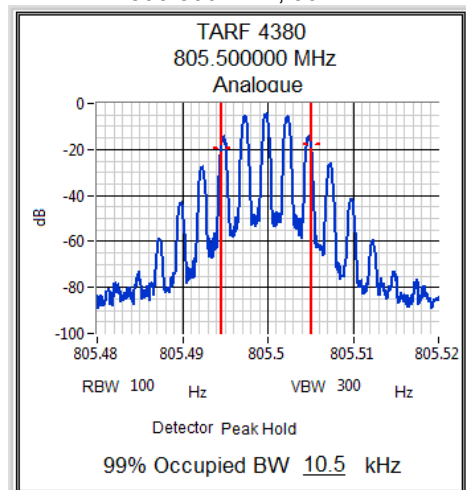
805.500 MHz, 30 W
