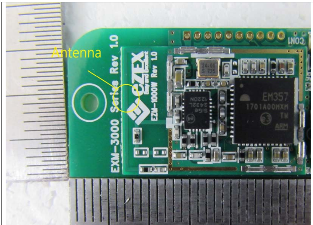
<Zigbee Antenna>
