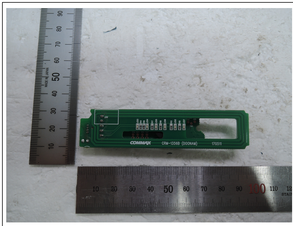
<Antenna>
