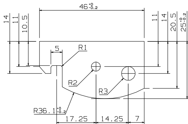
AH1 SERIAL 外形拔寸法図
