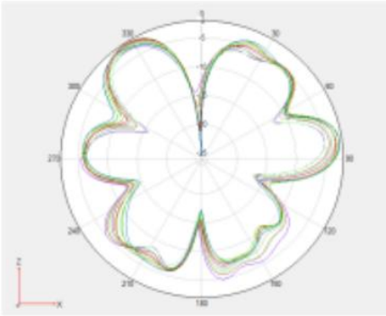
1950MHz Theta 90
