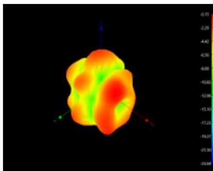
1950MHz Phi 90
