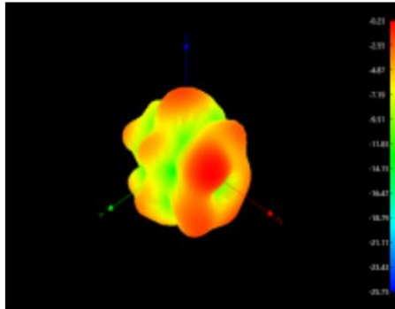
1900MHz Phi 90
