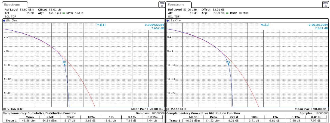
PAPR, TX 2155 MHz, BW: 5MHz, MOD: 256QAM
