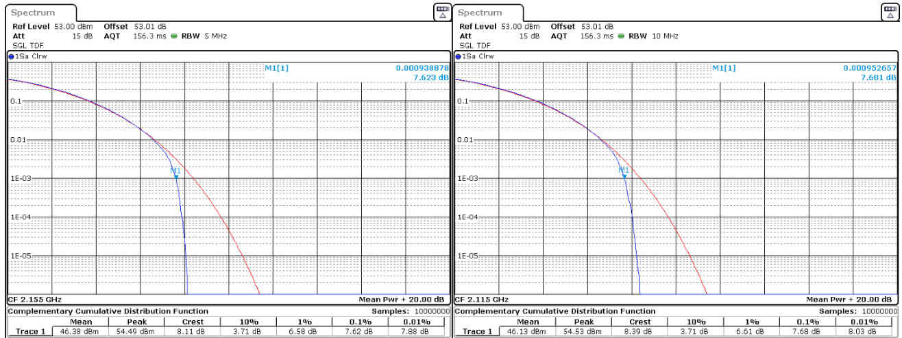
PAPR TX 2155 MHz, BW: 5MHz, MOD: 64QAM
