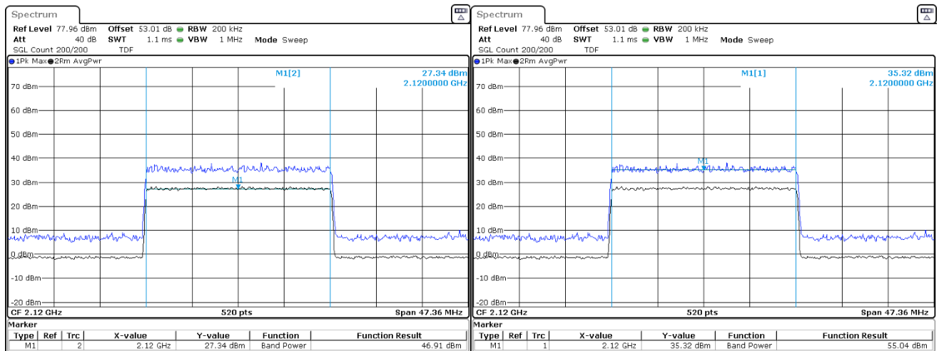
PAPR TX 2120 MHz, BW: 20MHz, MOD: 64QAM
