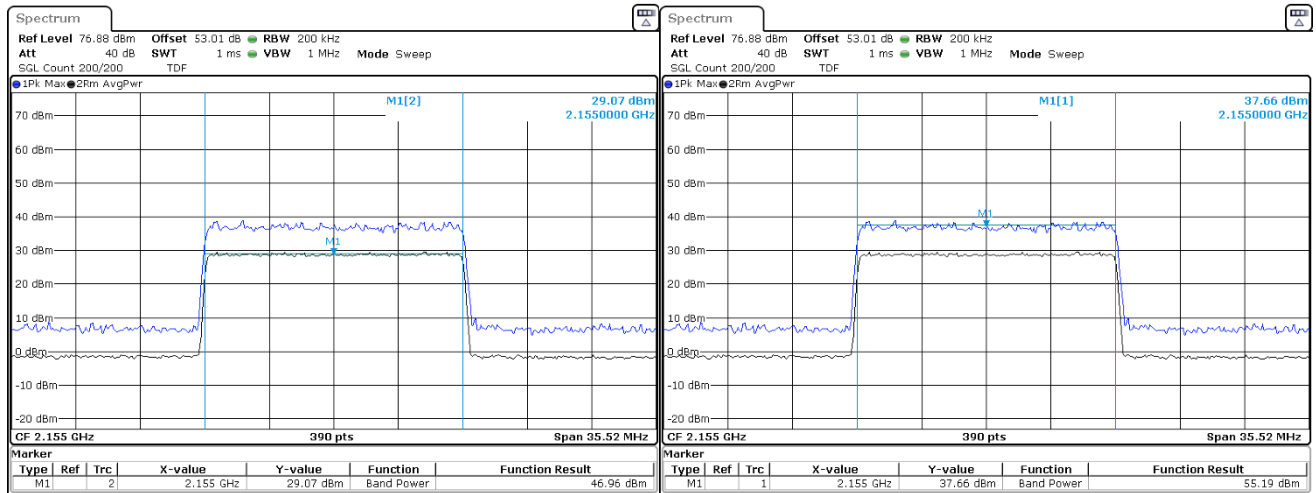
PAPR, TX 2155 MHz, BW: 15MHz, MOD: 256QAM
