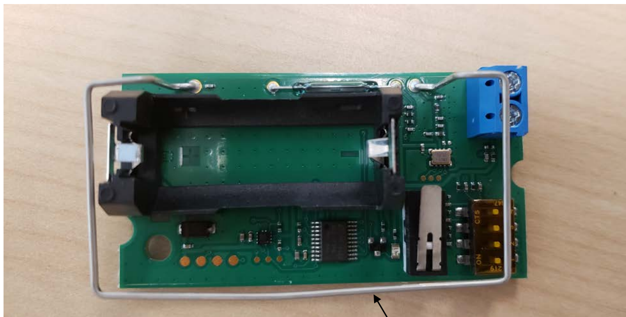
PCB TOP
